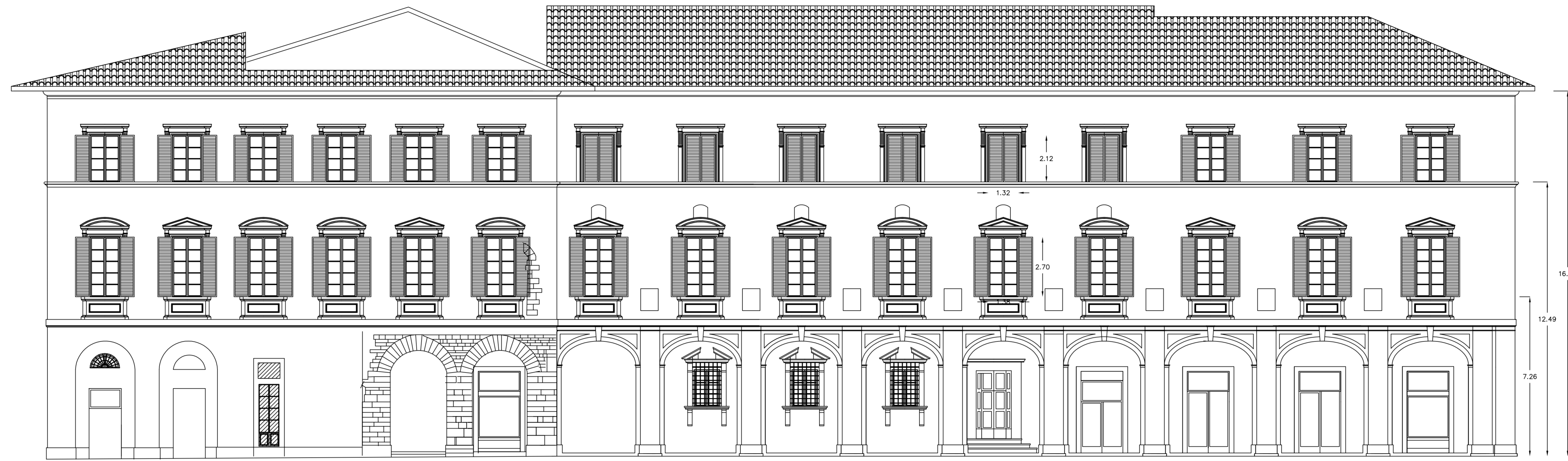
PROSPETTO VIA GUASTI – PIAZZA DEL COMUNE
