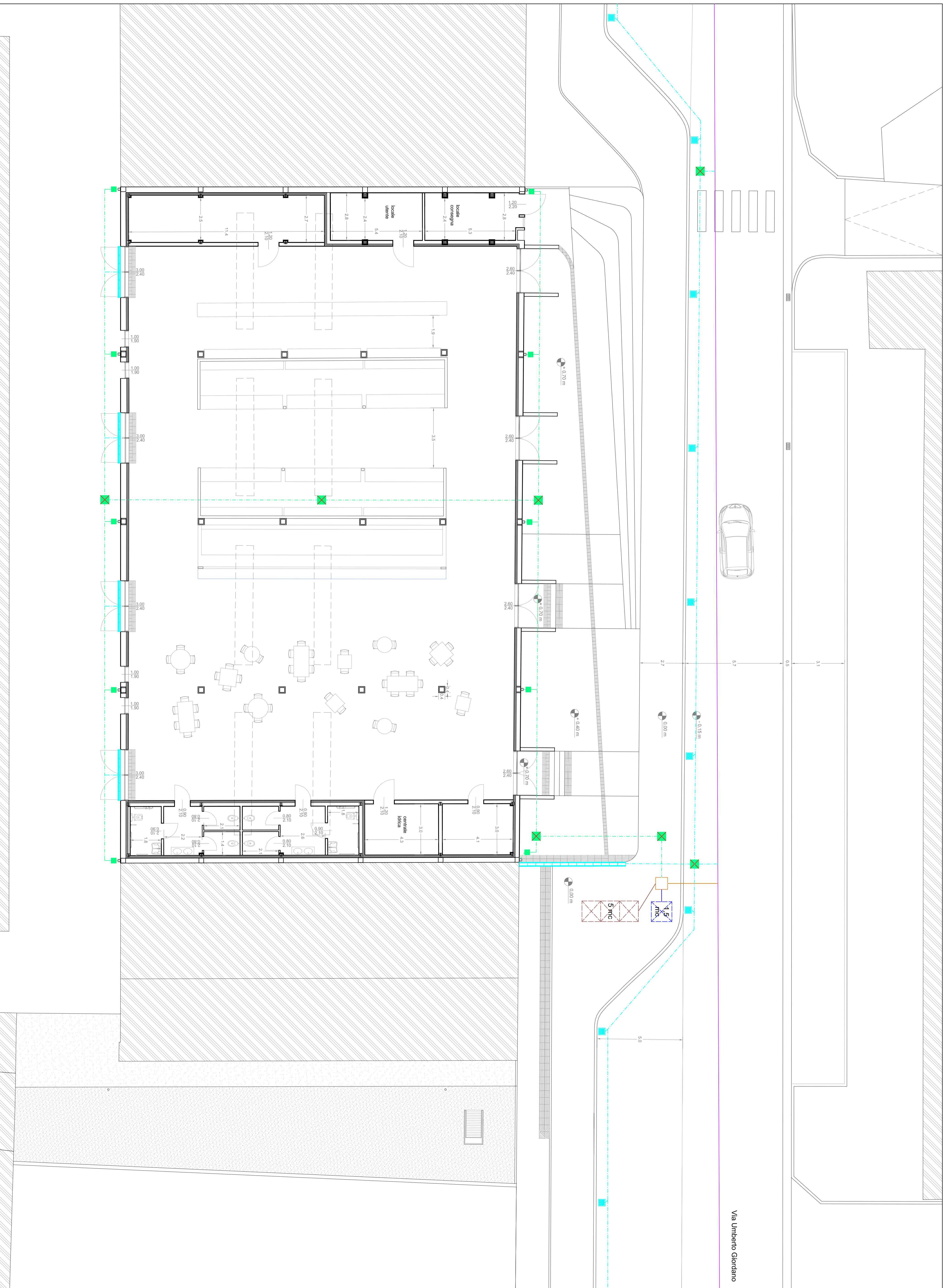
Planta Progetto rete di smaltimento. Scala 1:100
