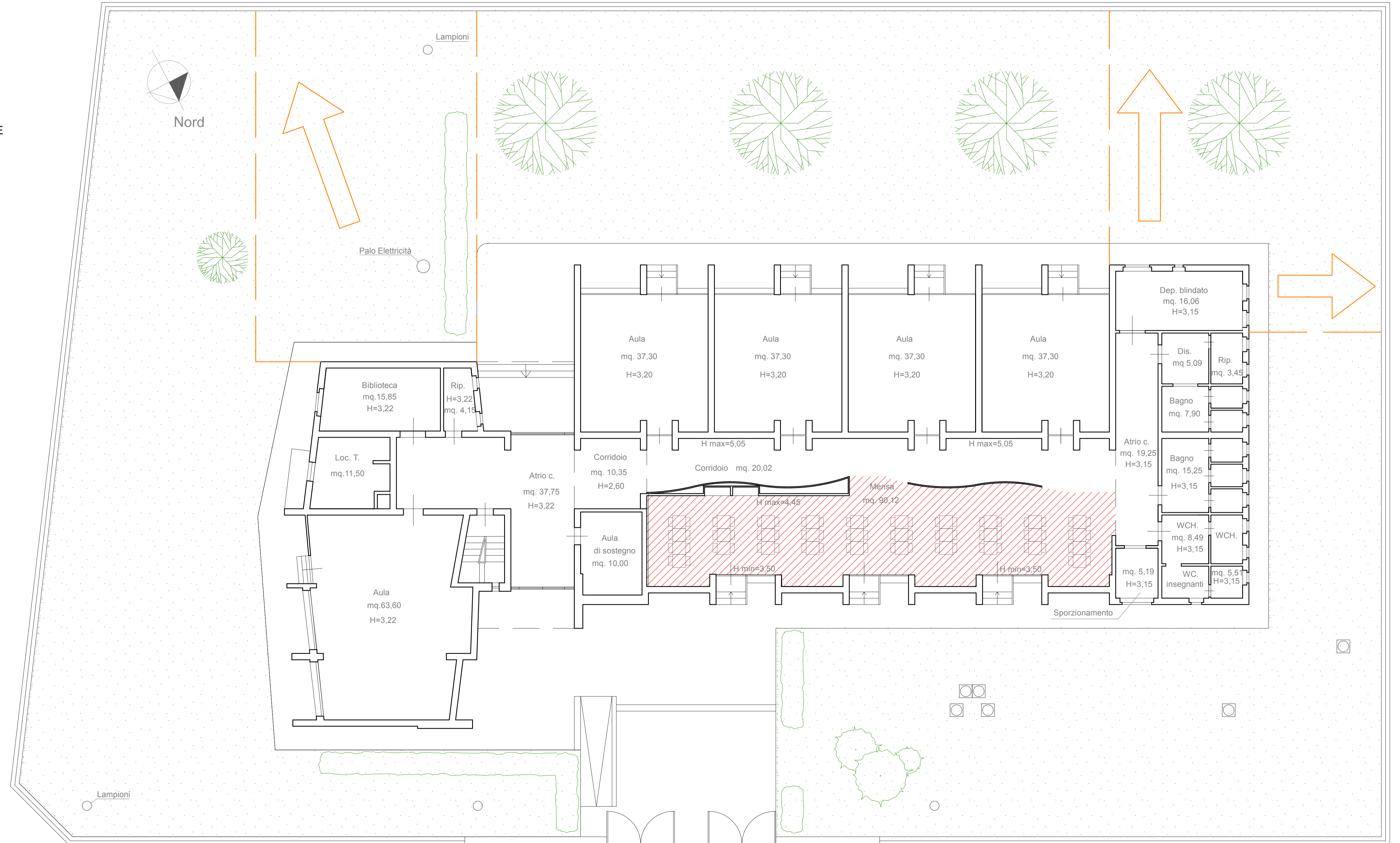
Pianta scuola primaria esistente "A. Bruni" con indicazione delle linee guida da seguire per la realizzazione del primo lotto - scala 1:100
