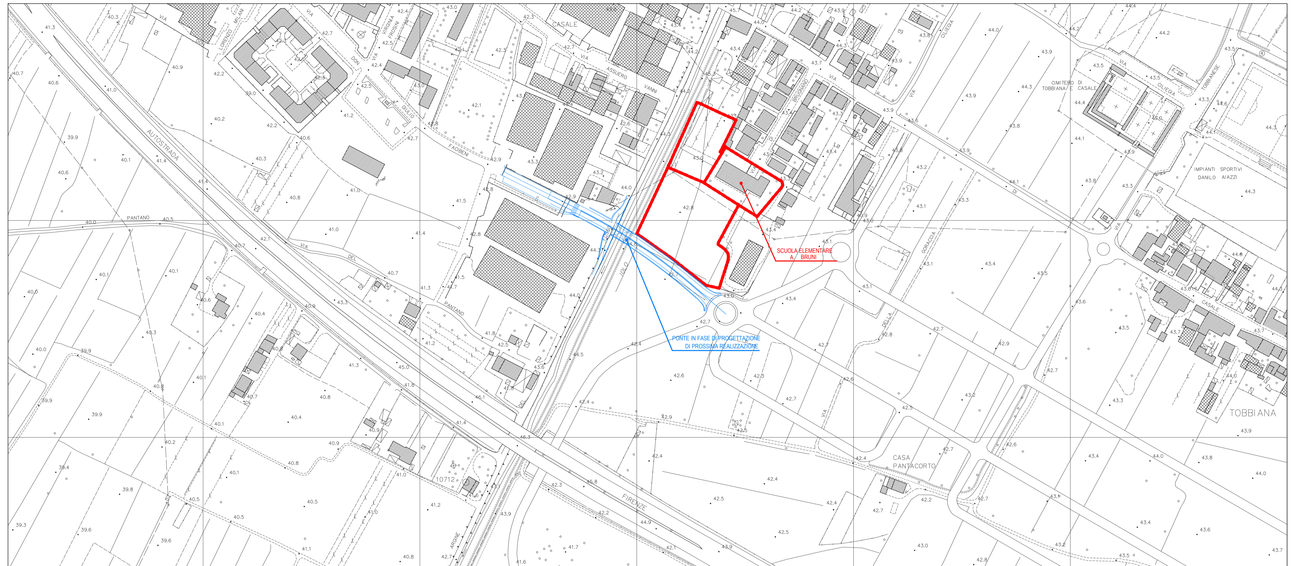
Planimetria Irtef con individuazione area di intervento - scala 1:2000
