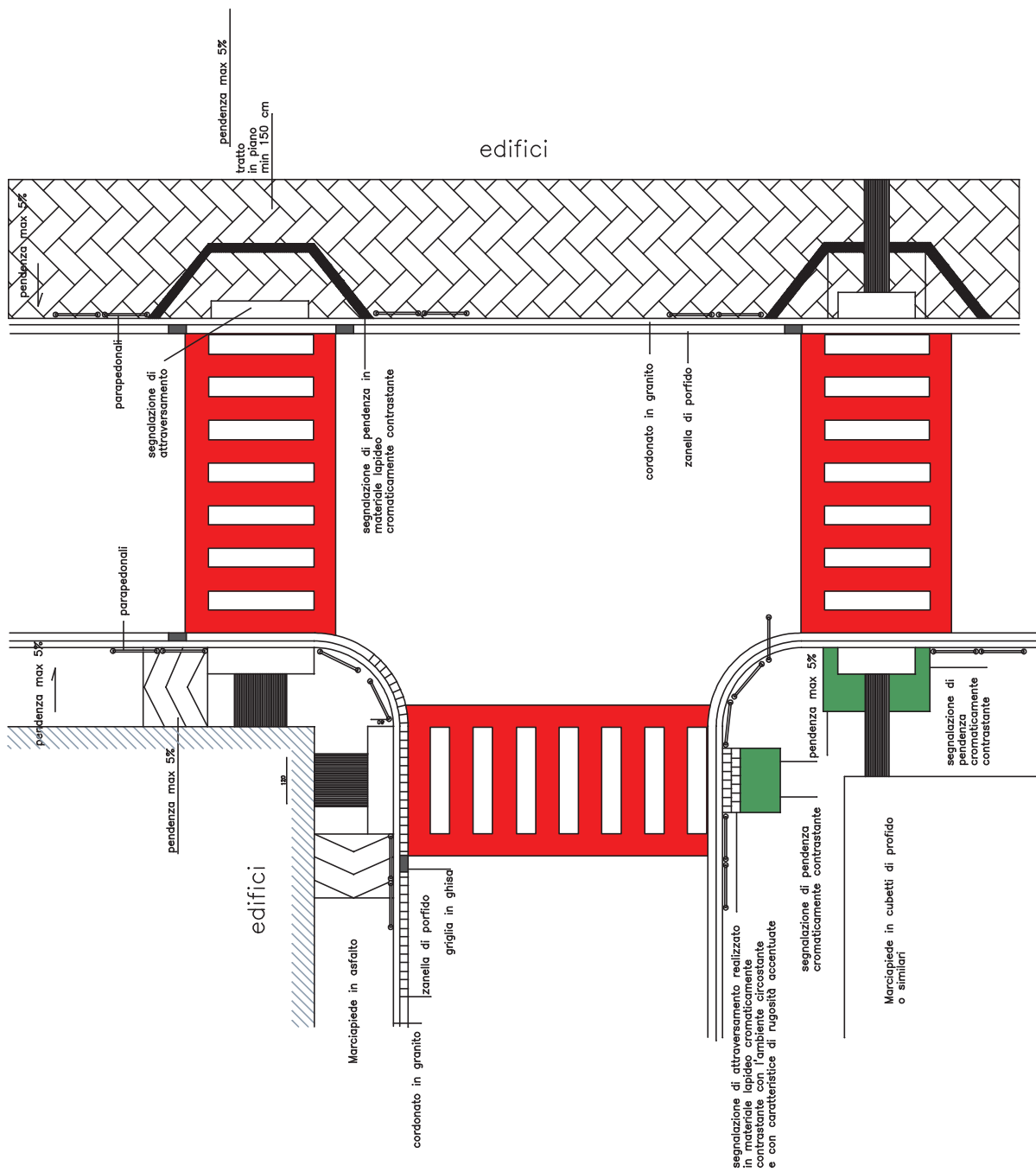
Schema tipo di attraversamenti pedonali in centro storico
