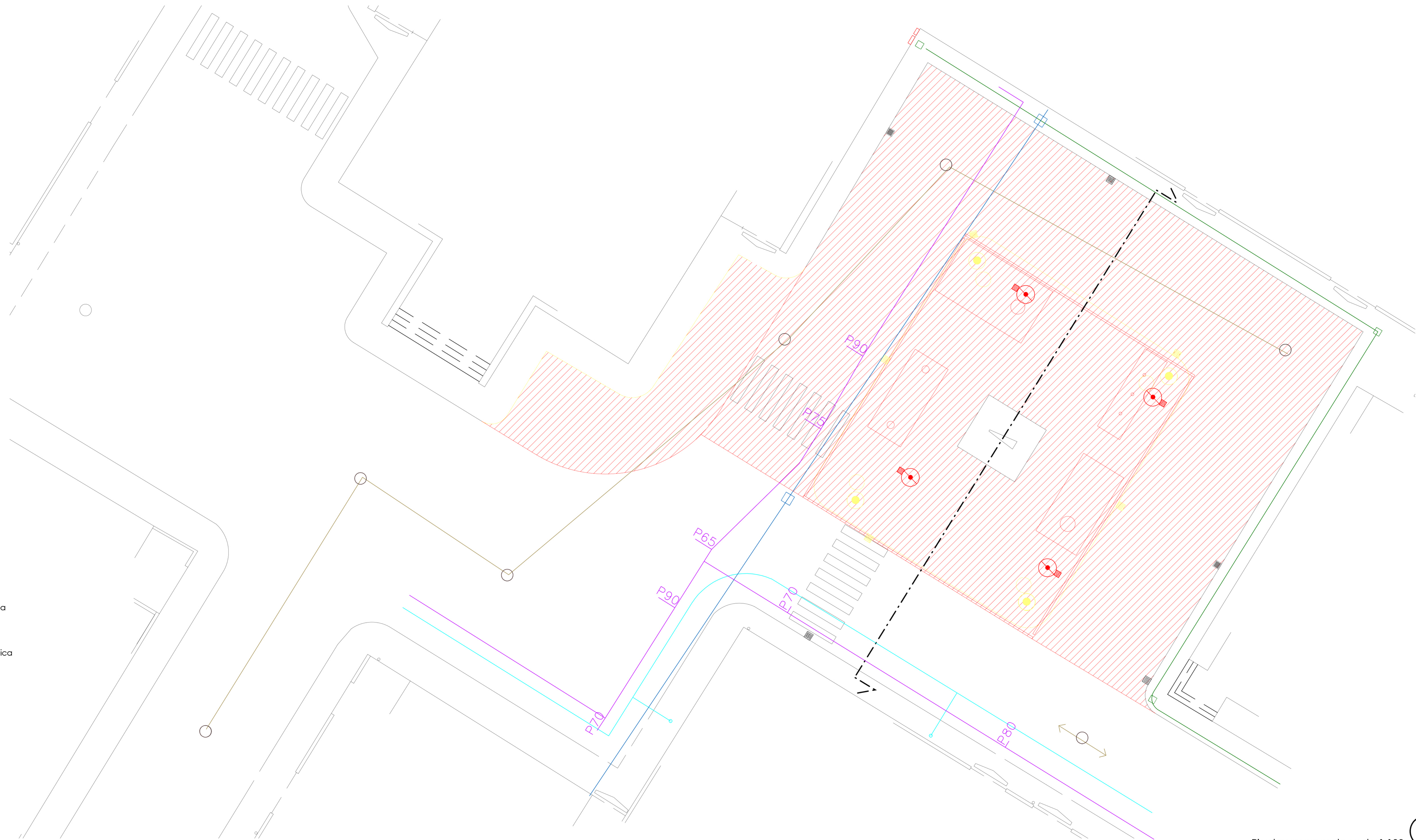
Pianta sovrapposto scala 1:100
