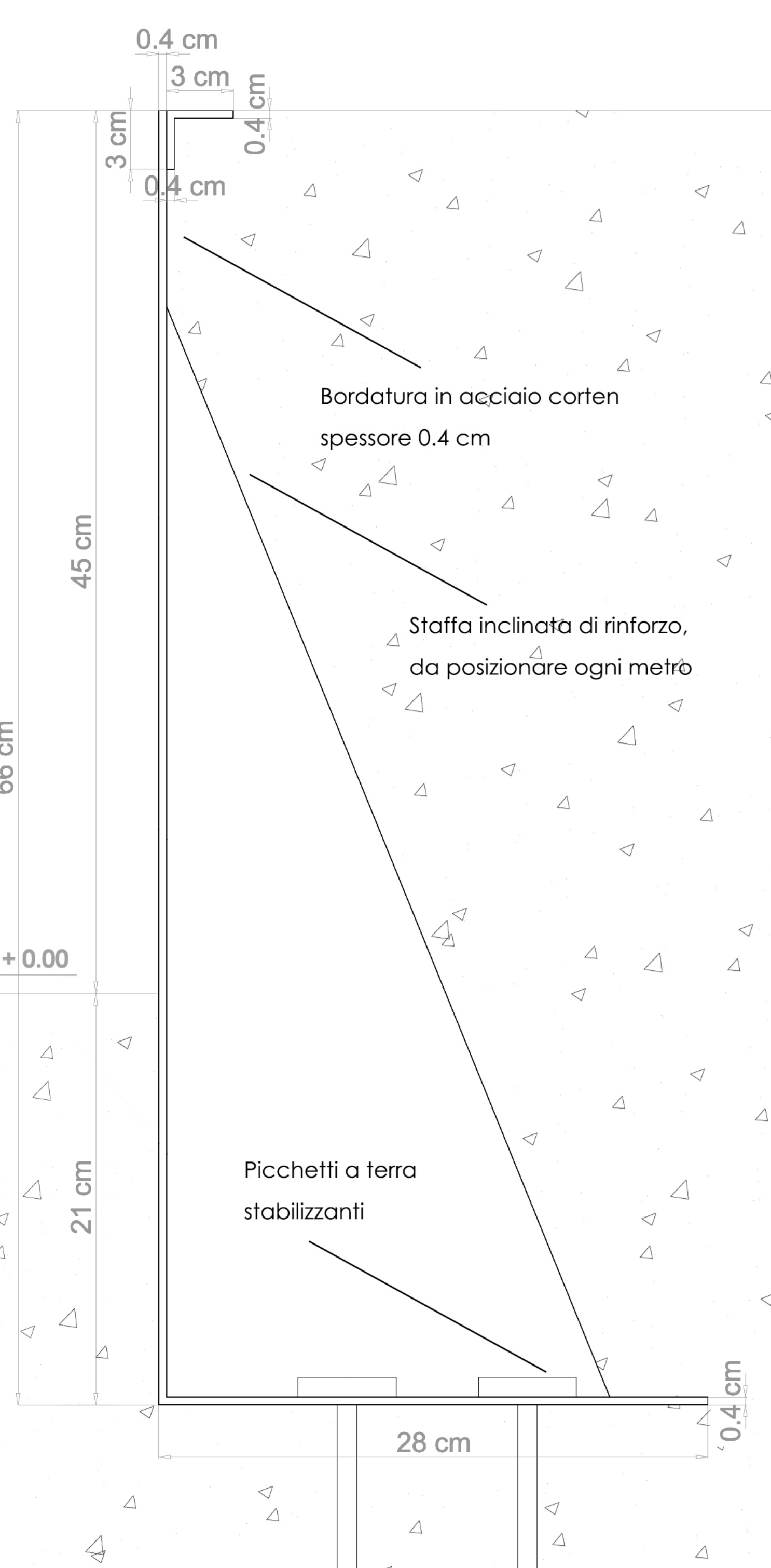
Particolare scala 1:20
