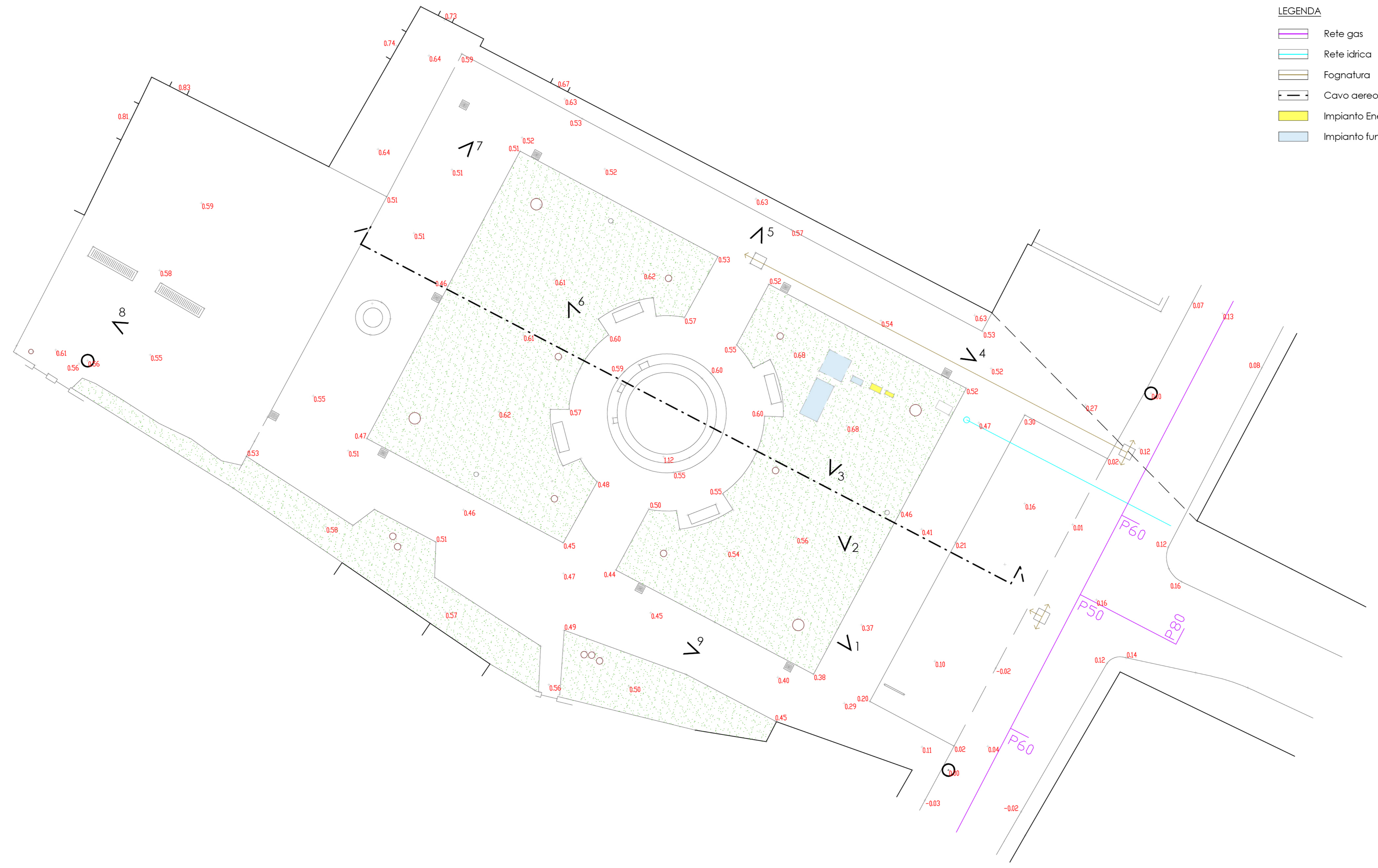
Pianta rilievo scala 1:100
