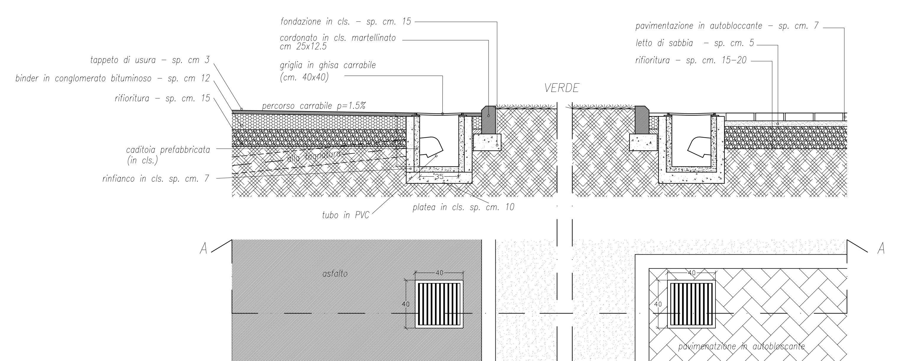
Particolare realizzazione pozzetto e cordonato
