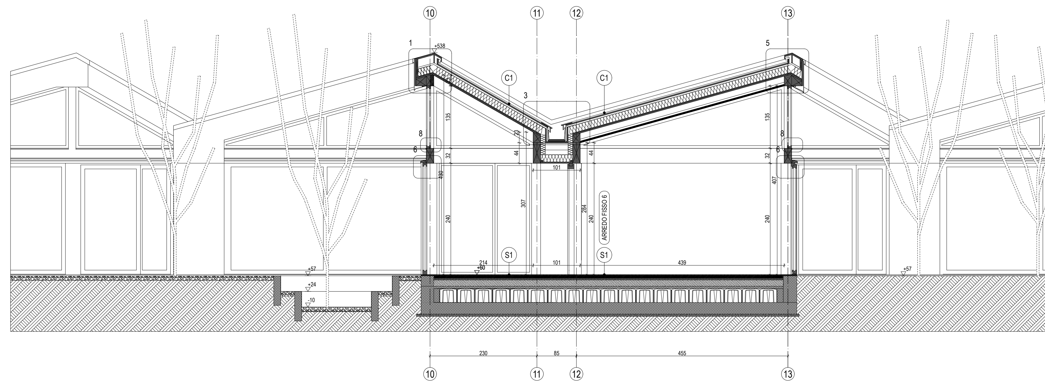
SEZIONE E
