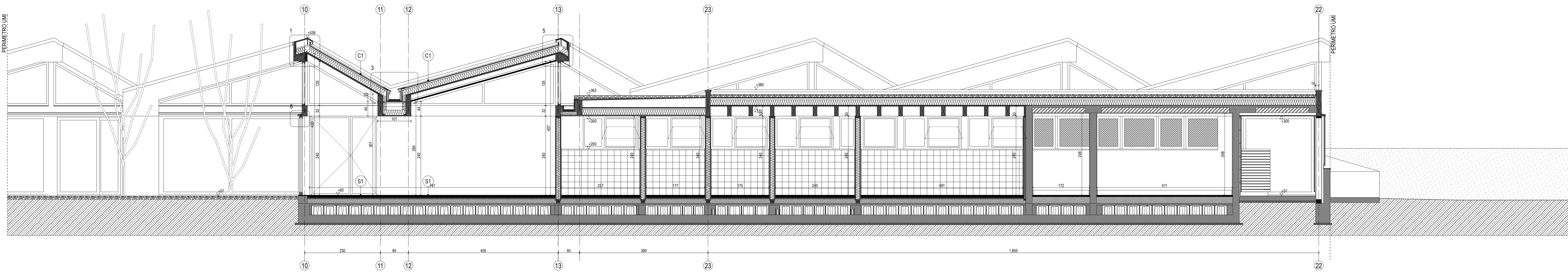
SEZIONE F
