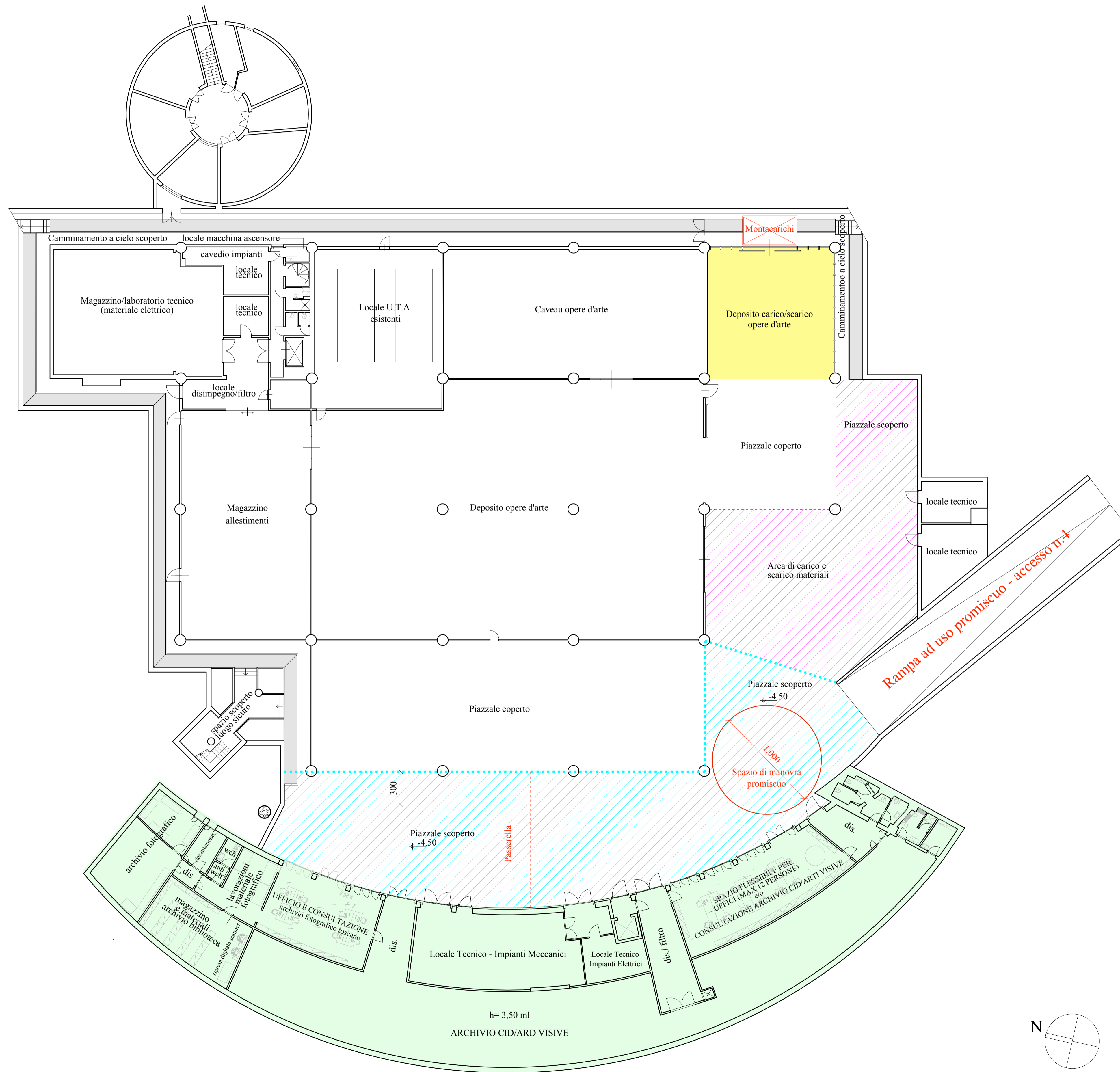
PIANTA PIANO INTERRATO
