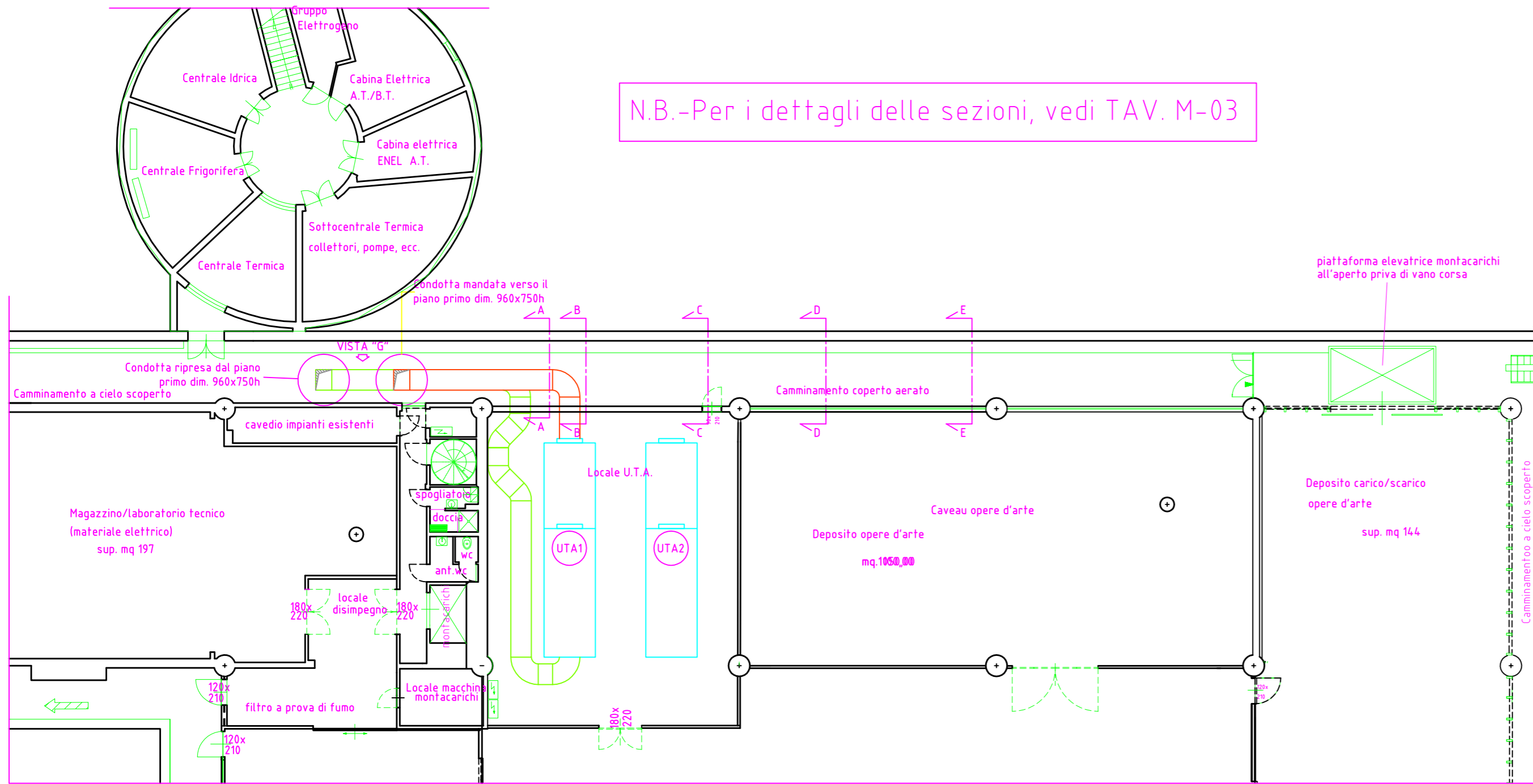
Passaggio canali scannafosso "UTA1"
