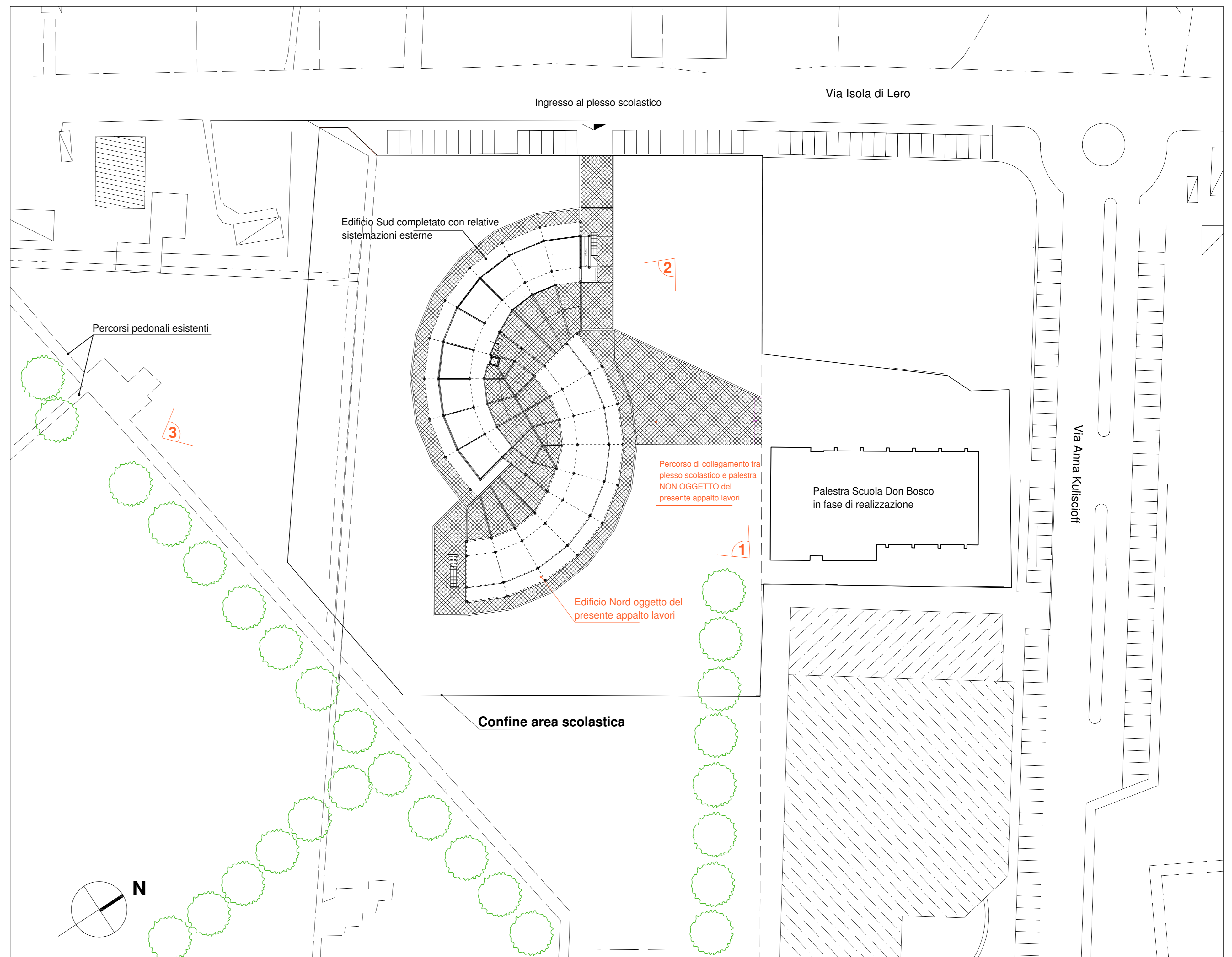
Inquadramento dell'area - stato di progetto, scala 1:500
