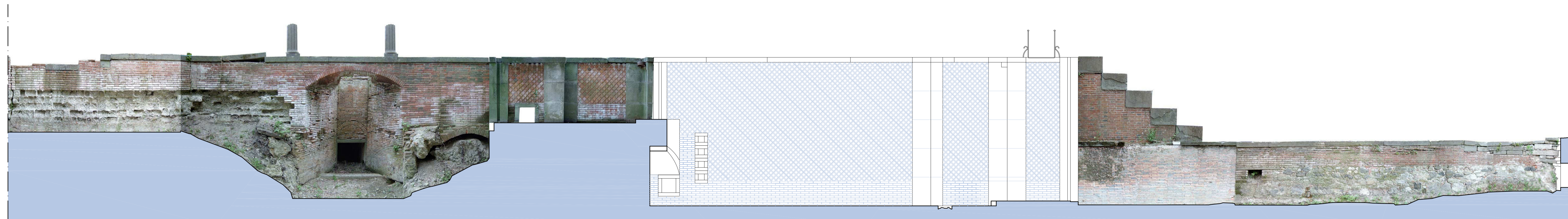
SEZIONE F-F' - Scala 1:50
