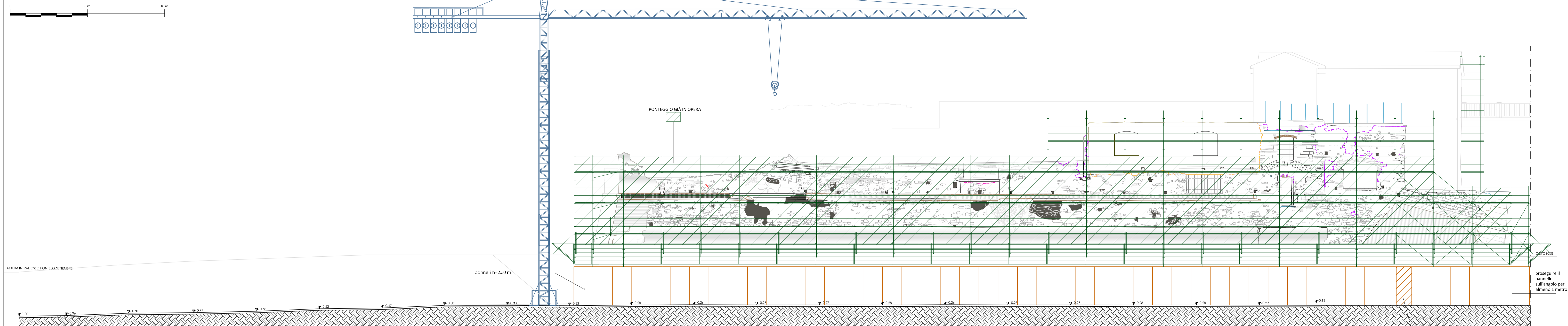
PROSPETTO DEI PONTEGGI FRONTE EST, Scala 1:100
