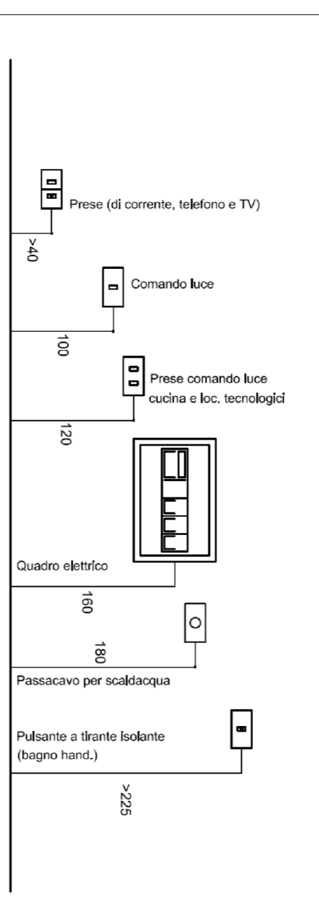
Quote di installazione
