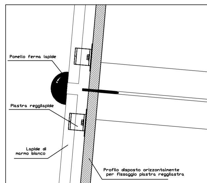
Particolare fissaggio lapide, Scala 1:20
