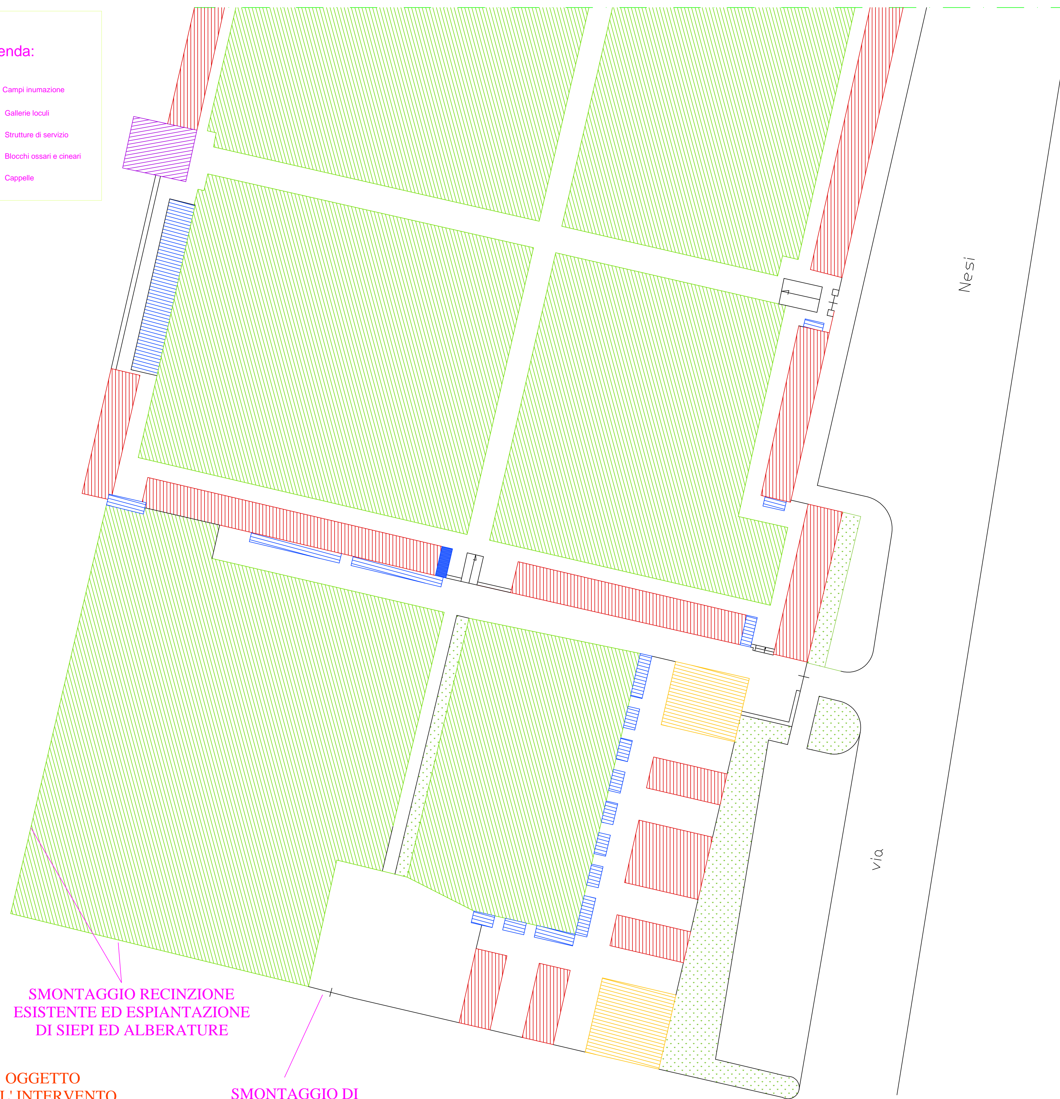
Planimetria generale, scala 1:200
