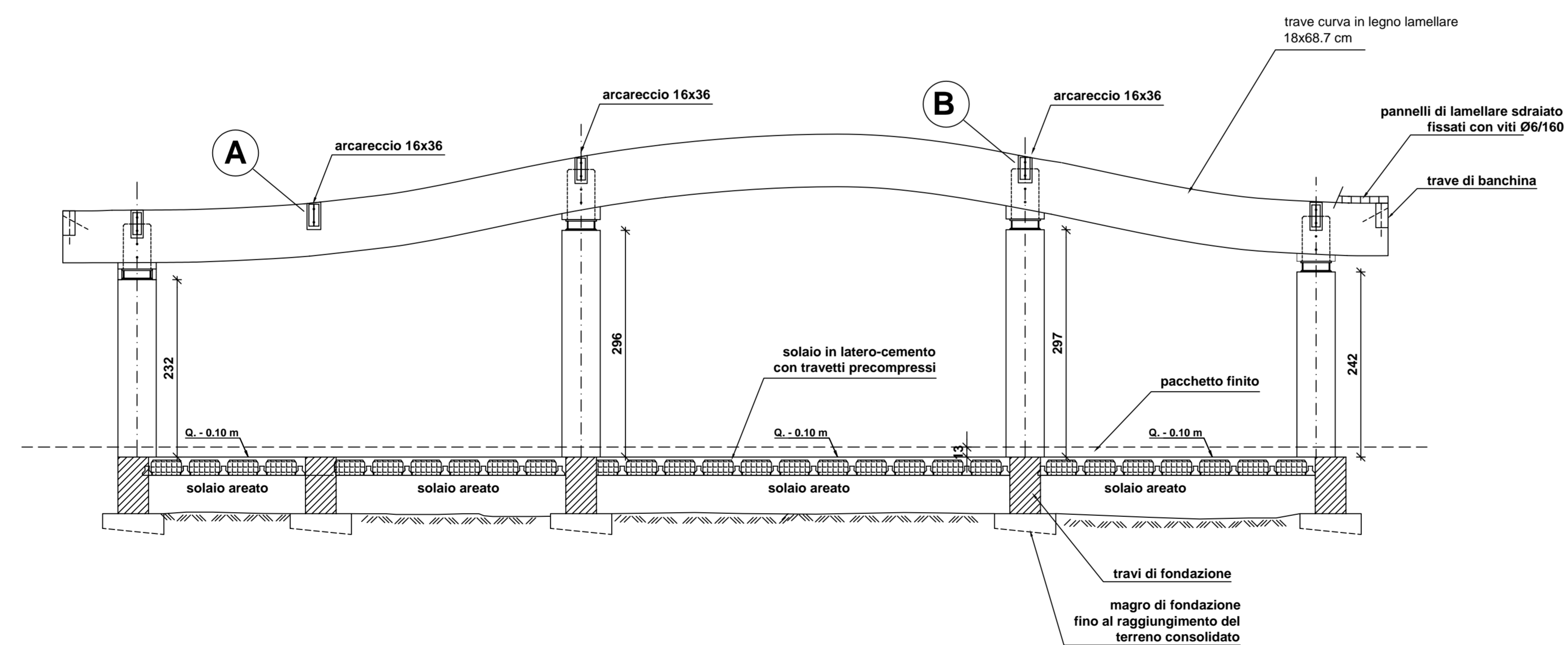
SEZIONE A-A
