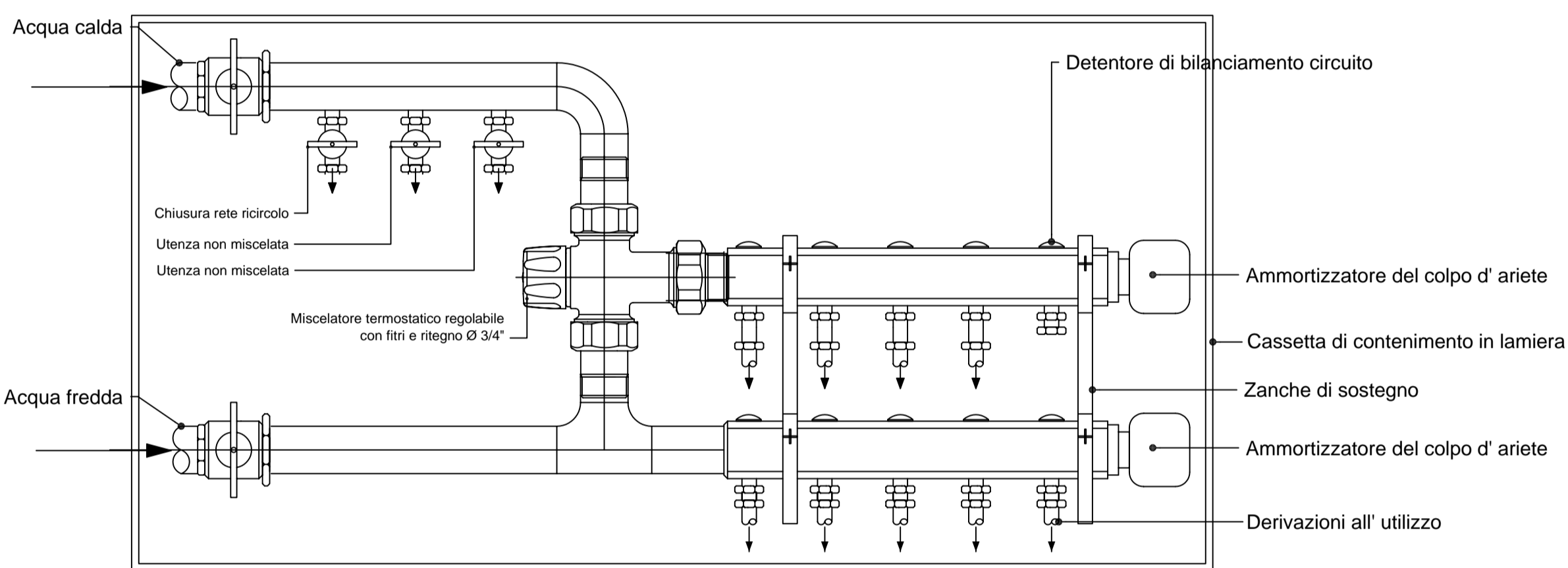
Particolare collettore distributore sanitario Particolare schematico, non in scala
