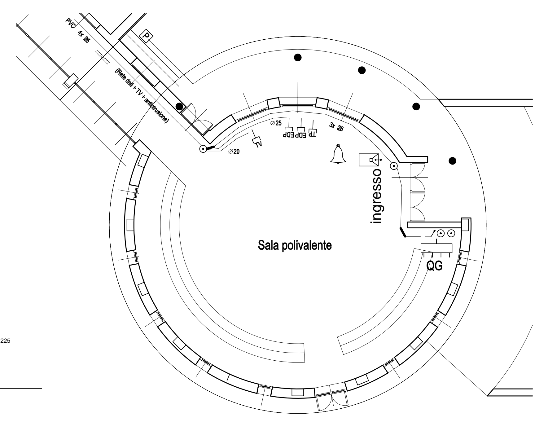
Impianti Speciali Distribuzione generale interna PIANO TERRA scala 1:100
