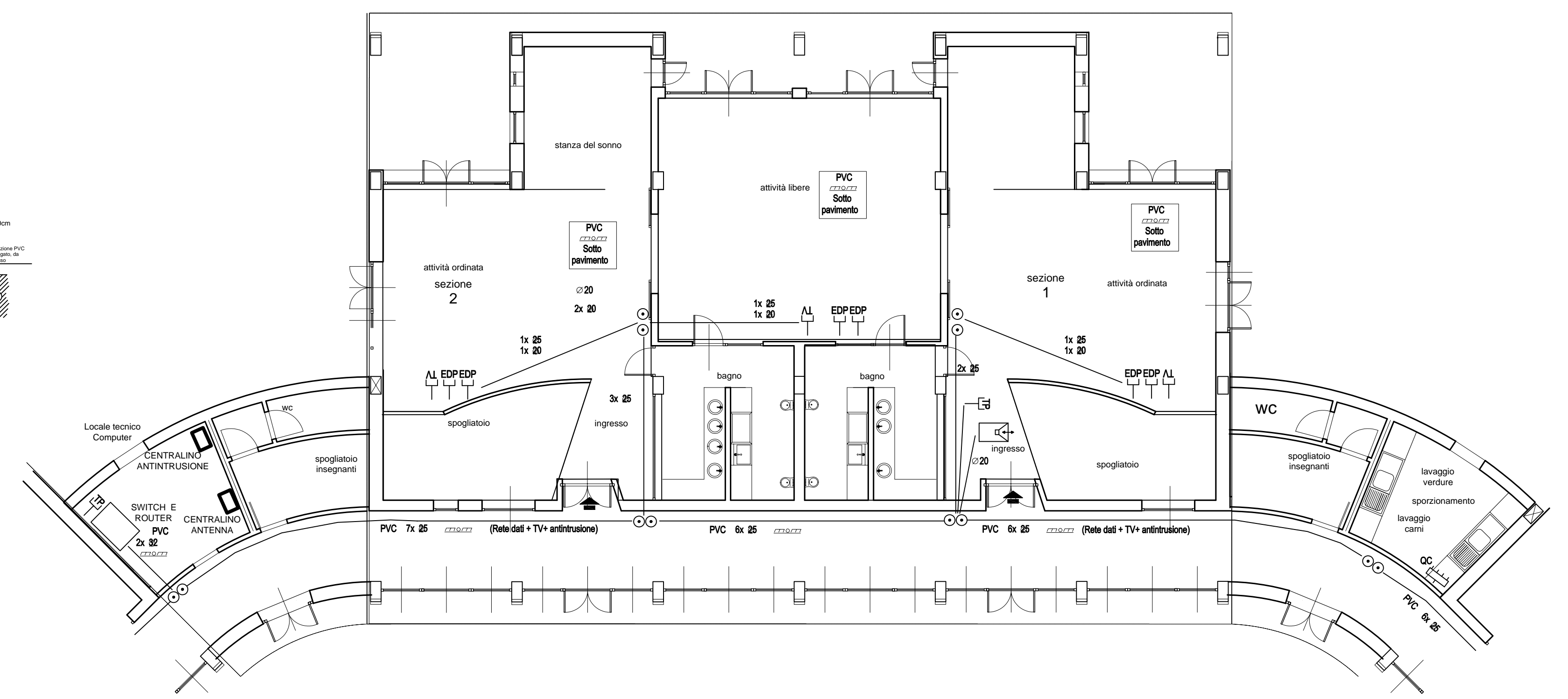
Impianti Speciali Distribuzione generale interna PIANO TERRA scala 1:100
