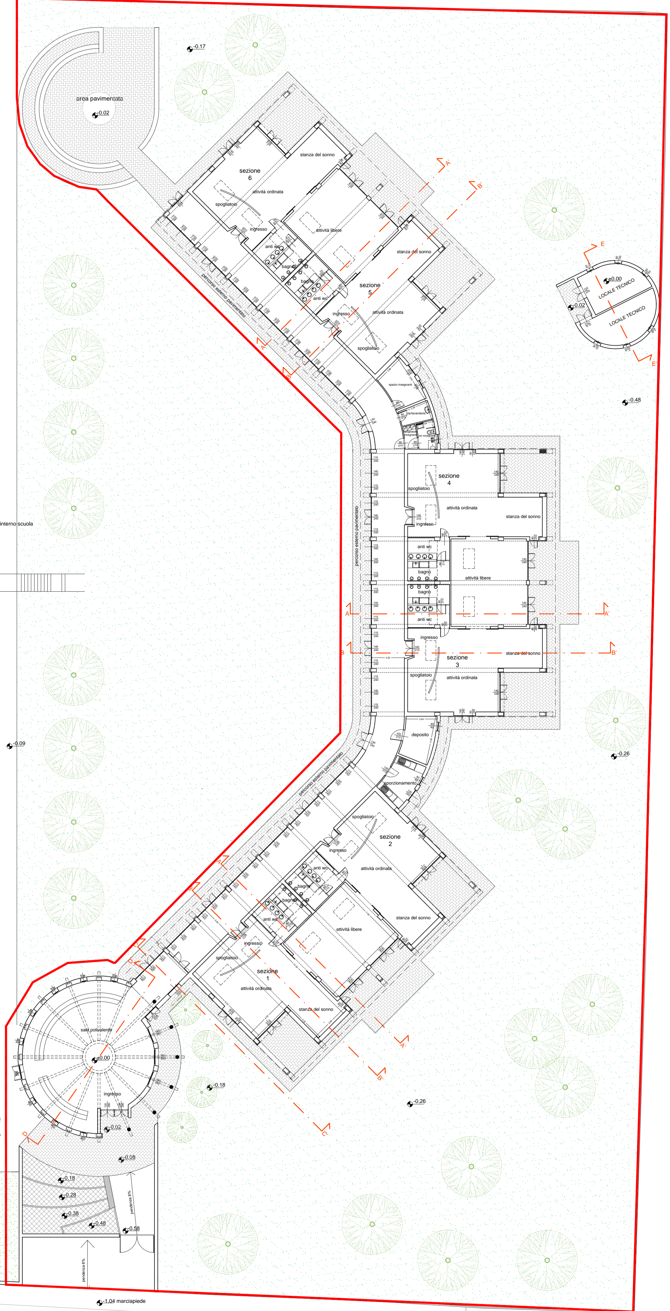
Pianta del complesso scolastico Scala 1/200
