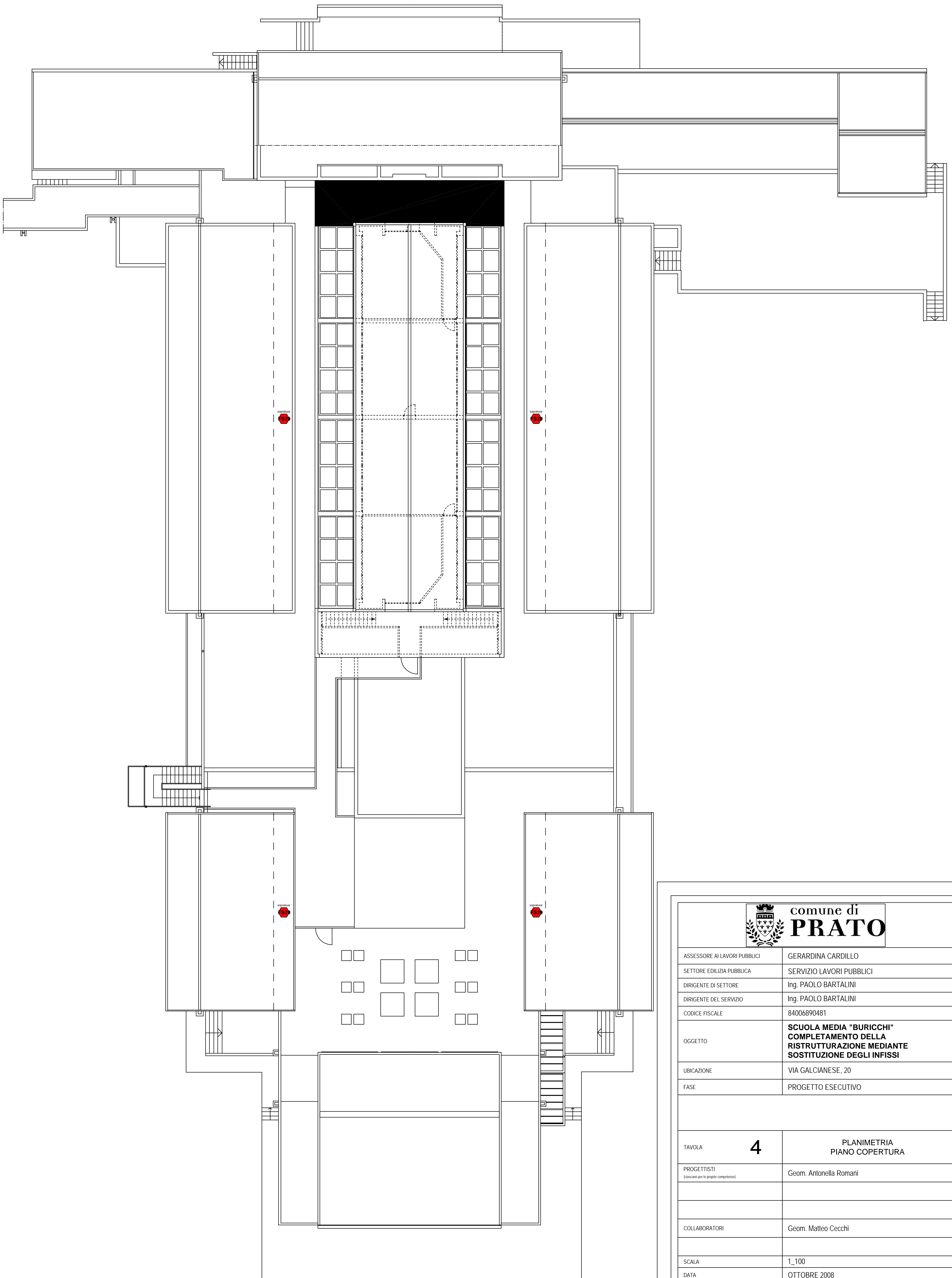
PIANTA PIANO COPERTURA — scala 1:100
