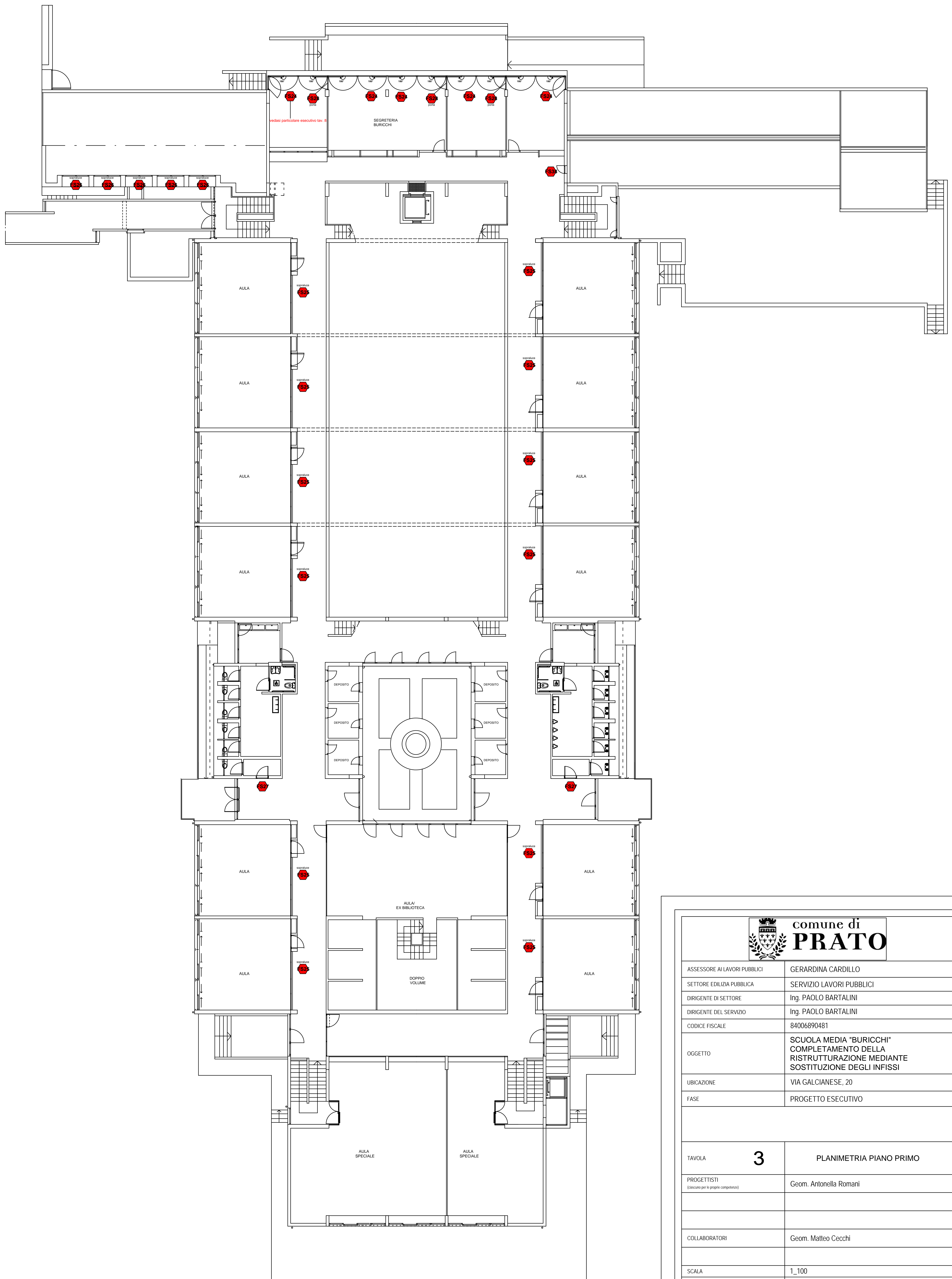
PIANTA PIANO PRIMO - scala 1:100
