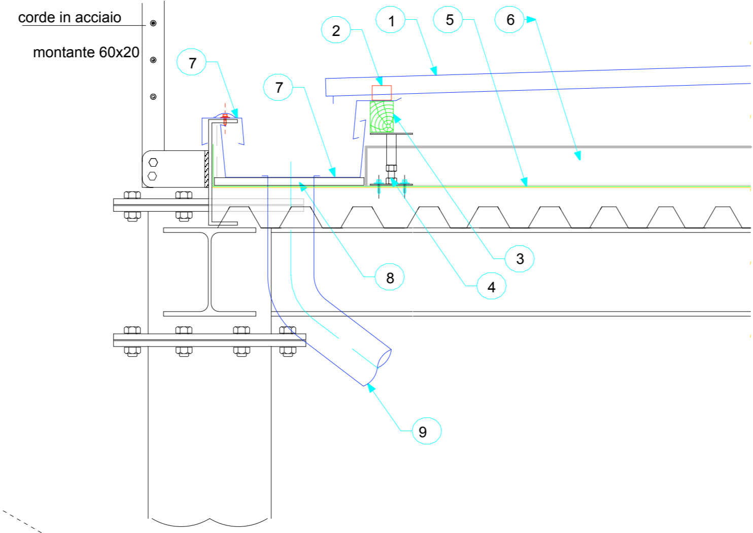
PARTICOLARE 1 CANALE DI GRONDA LATERALE
