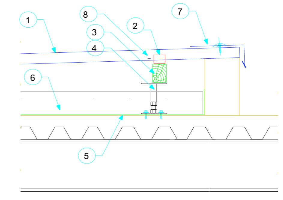
PARTICOLARE 3 RACCORDO CON MURO DEI CAMMINAMENTI
