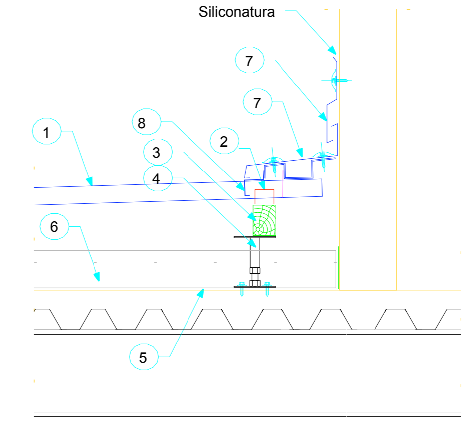
PARTICOLARE 2 RACCORDO CON MURO CENTRALE TERMICA E CAMMINAMENTI
