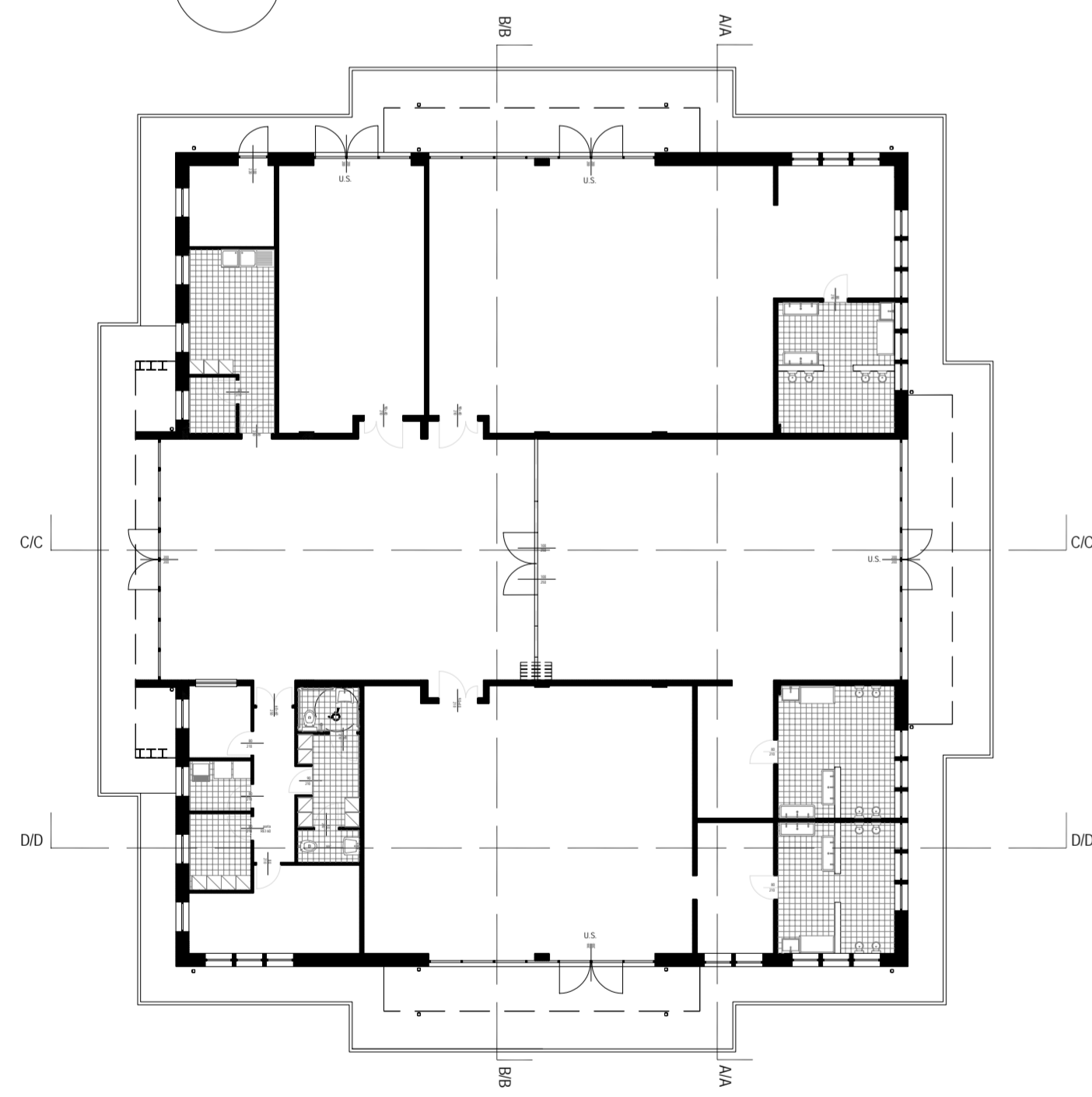
planimetria generale 1/200
