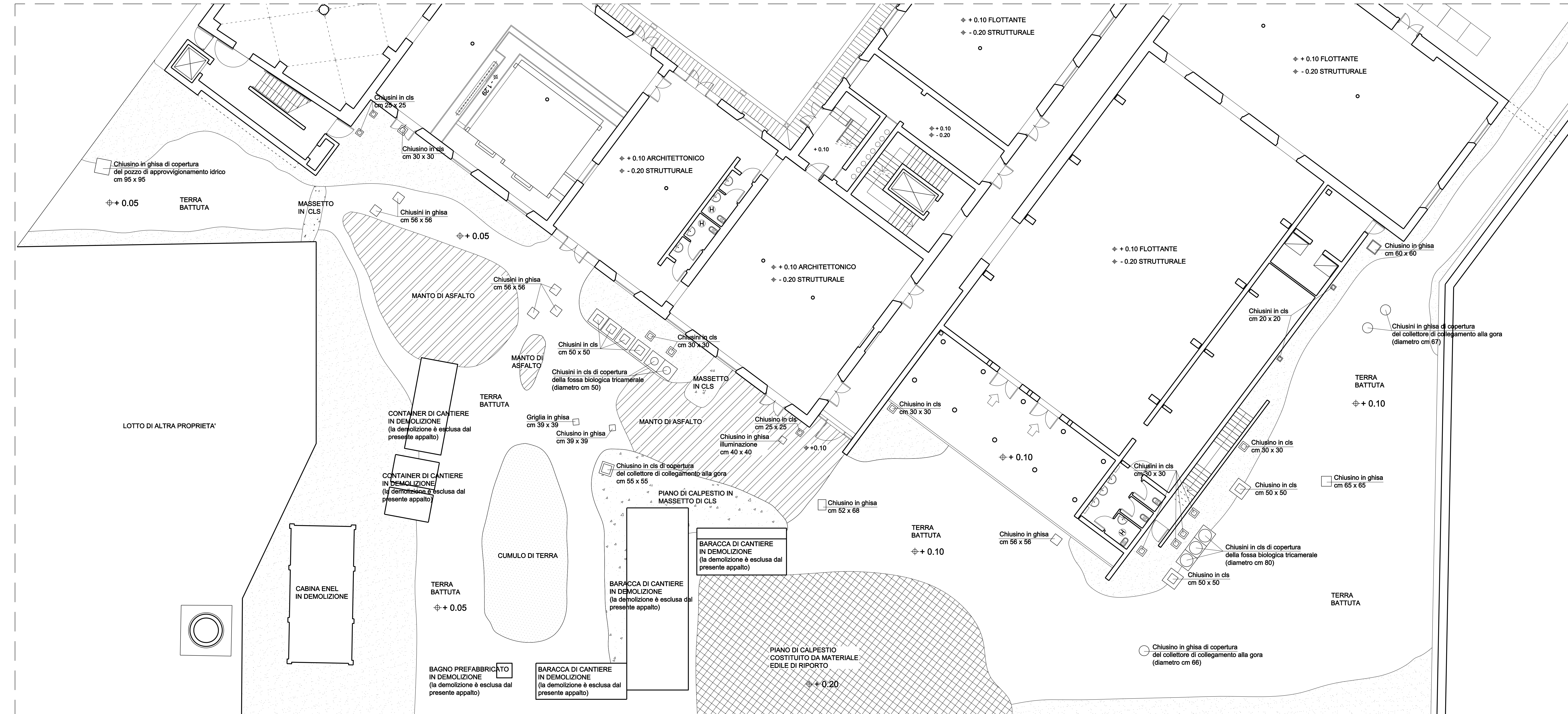
PIANTA PIAZZA DELLE MURA URBANE Scala 1:100
