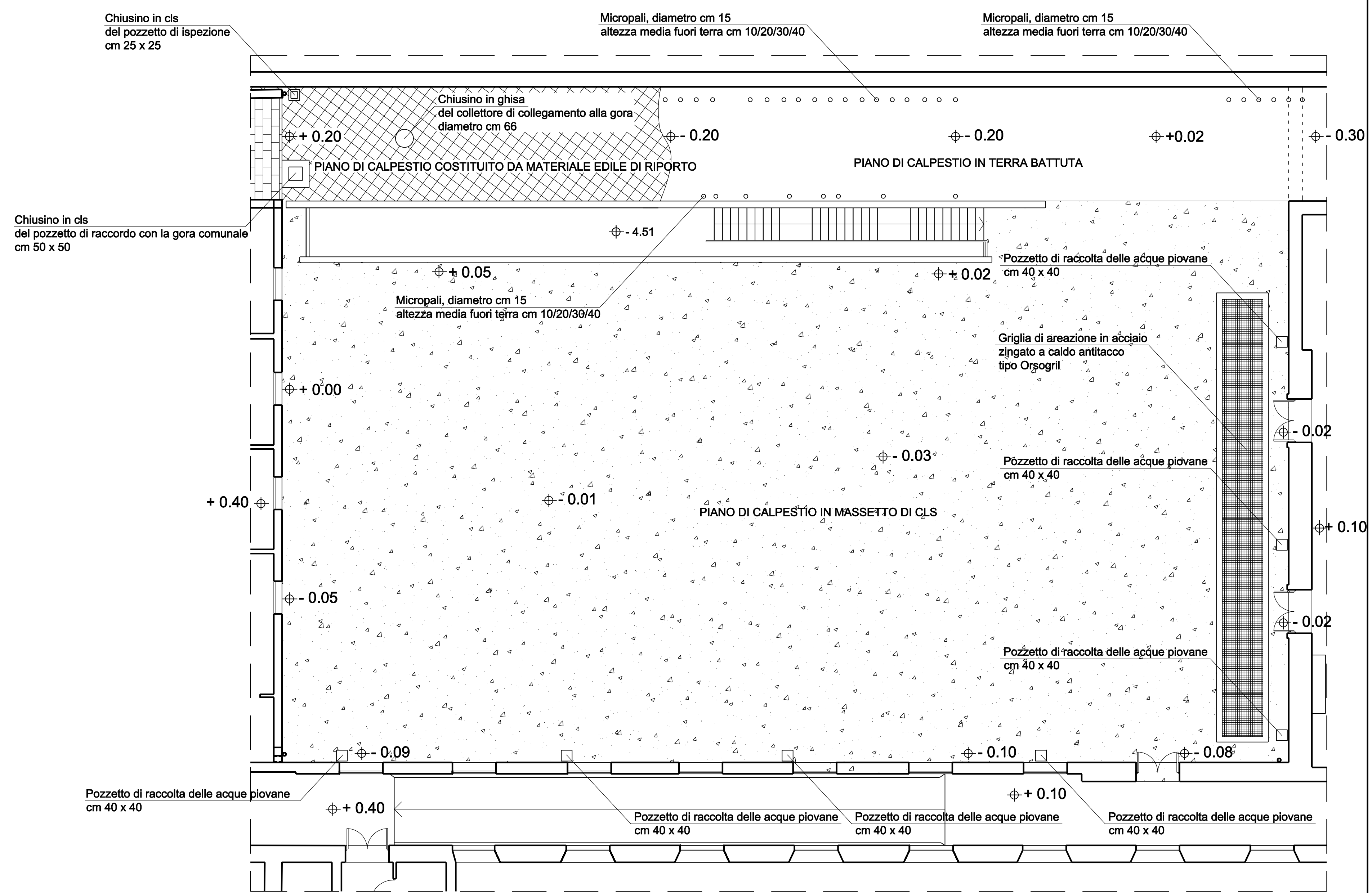
PIANTA CORTE DELLE SCULTURE Scala 1:100
