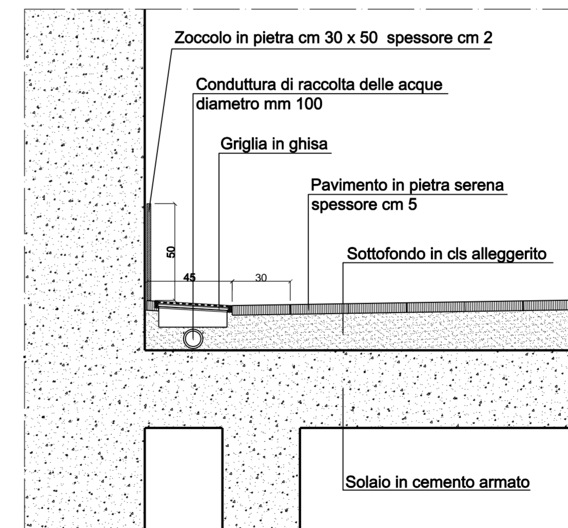
Particolare Sezione Scala 1:20
