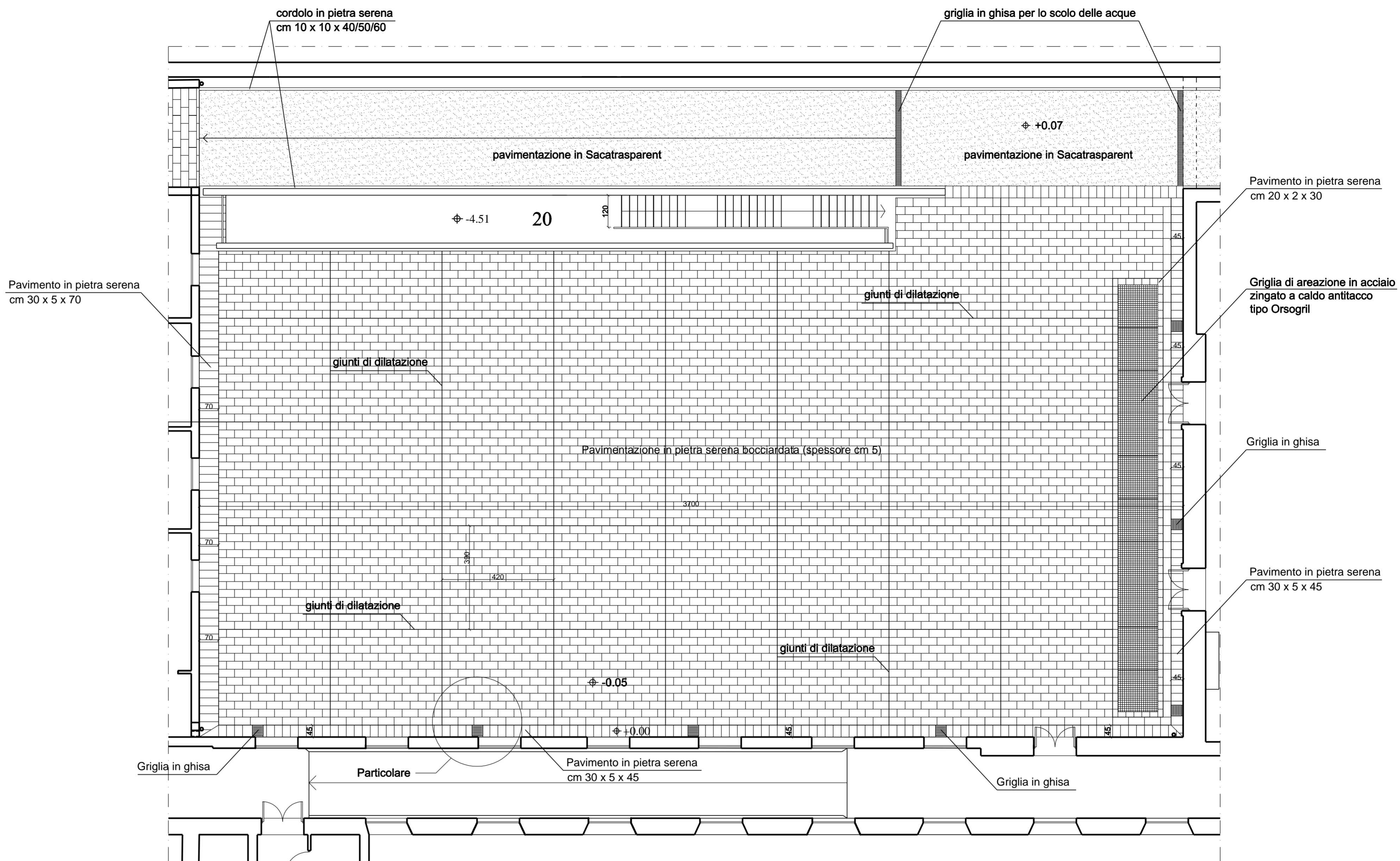
PIANTA CORTE DELLE SCULTURE Scala 1:100
