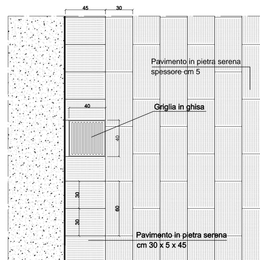
Particolare Pianta Scala 1:20
