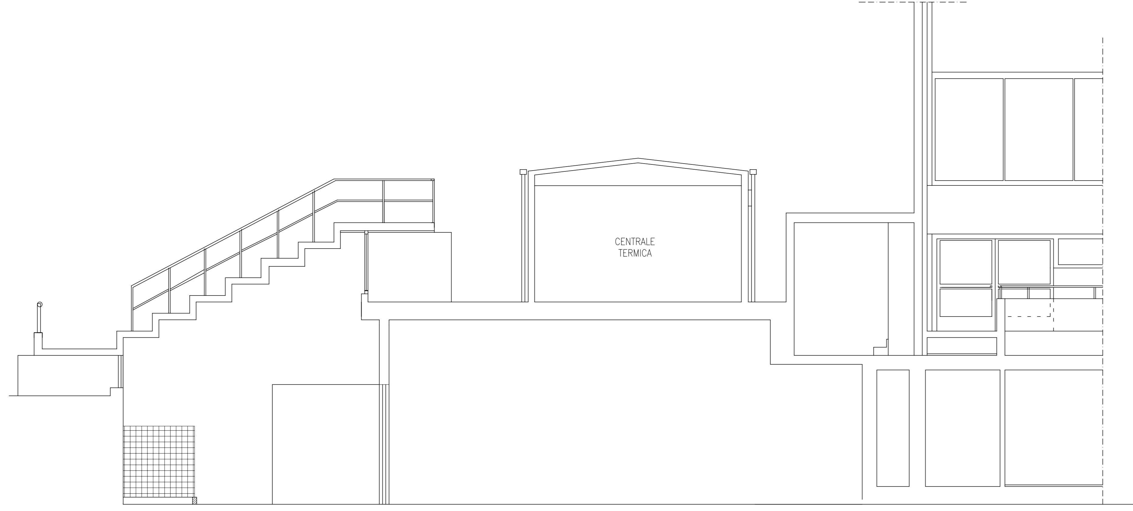
SEZ. A-A
