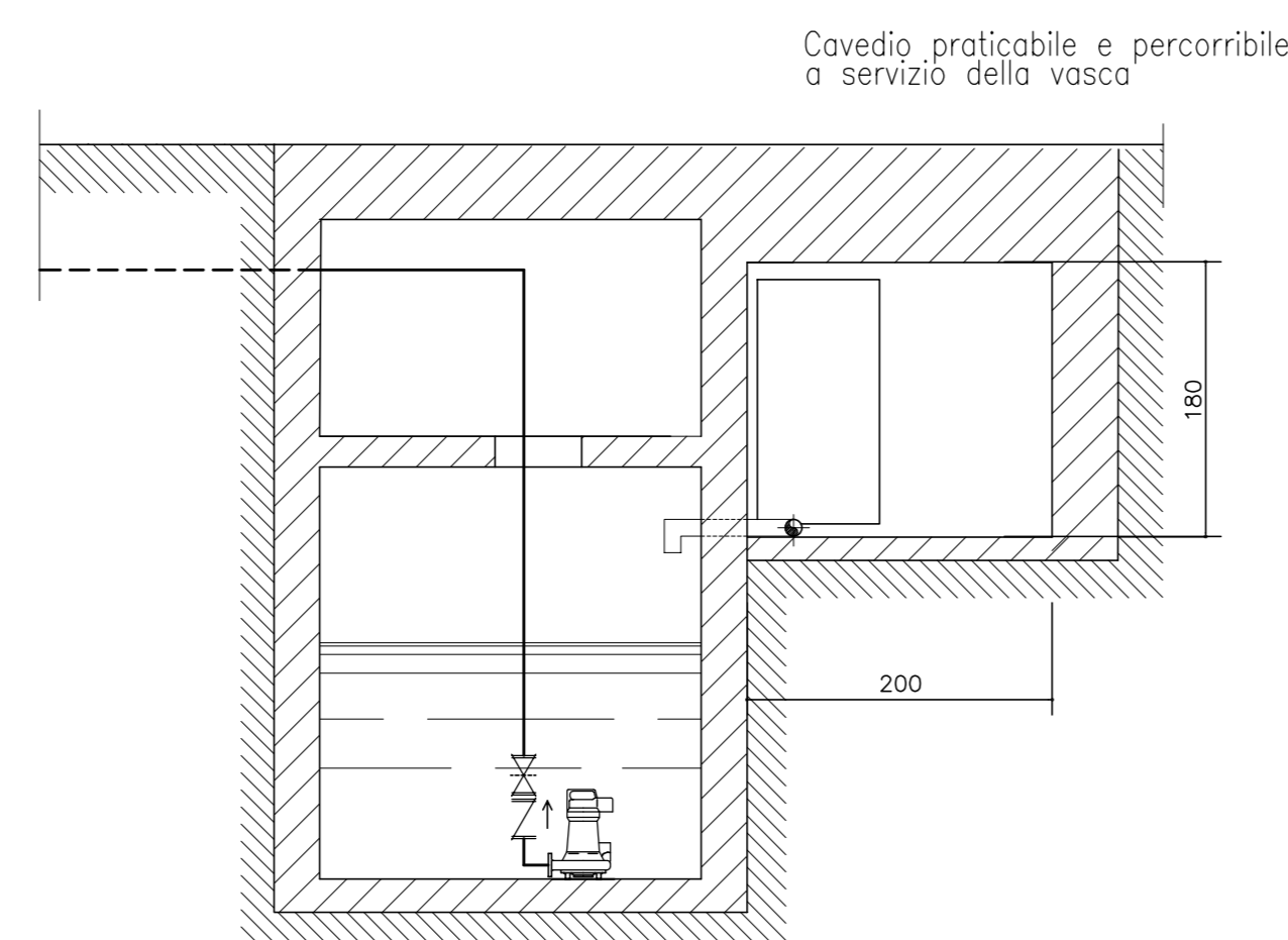
SEZ. E-E
