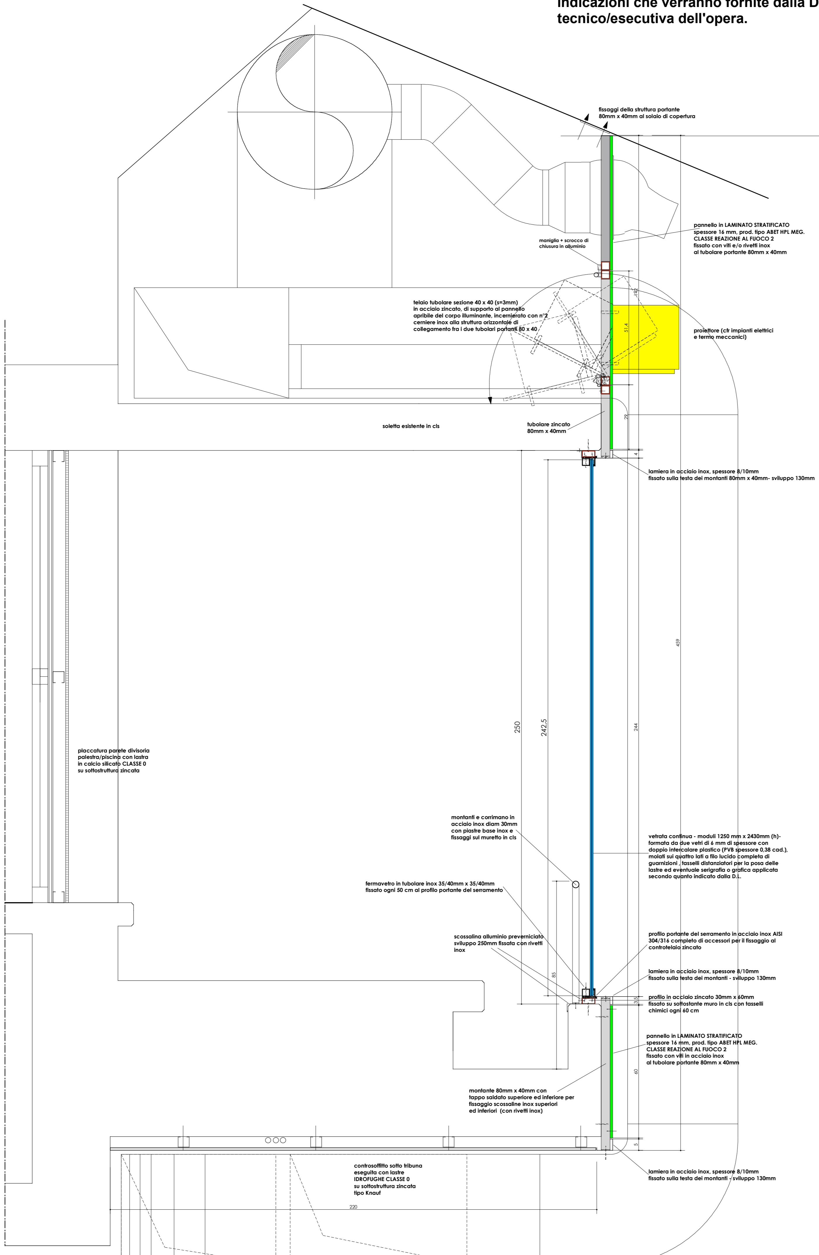
TRIBUNA SPETTATORI PISCINA - SEZIONE TRASVERSALE - scala 1/10
