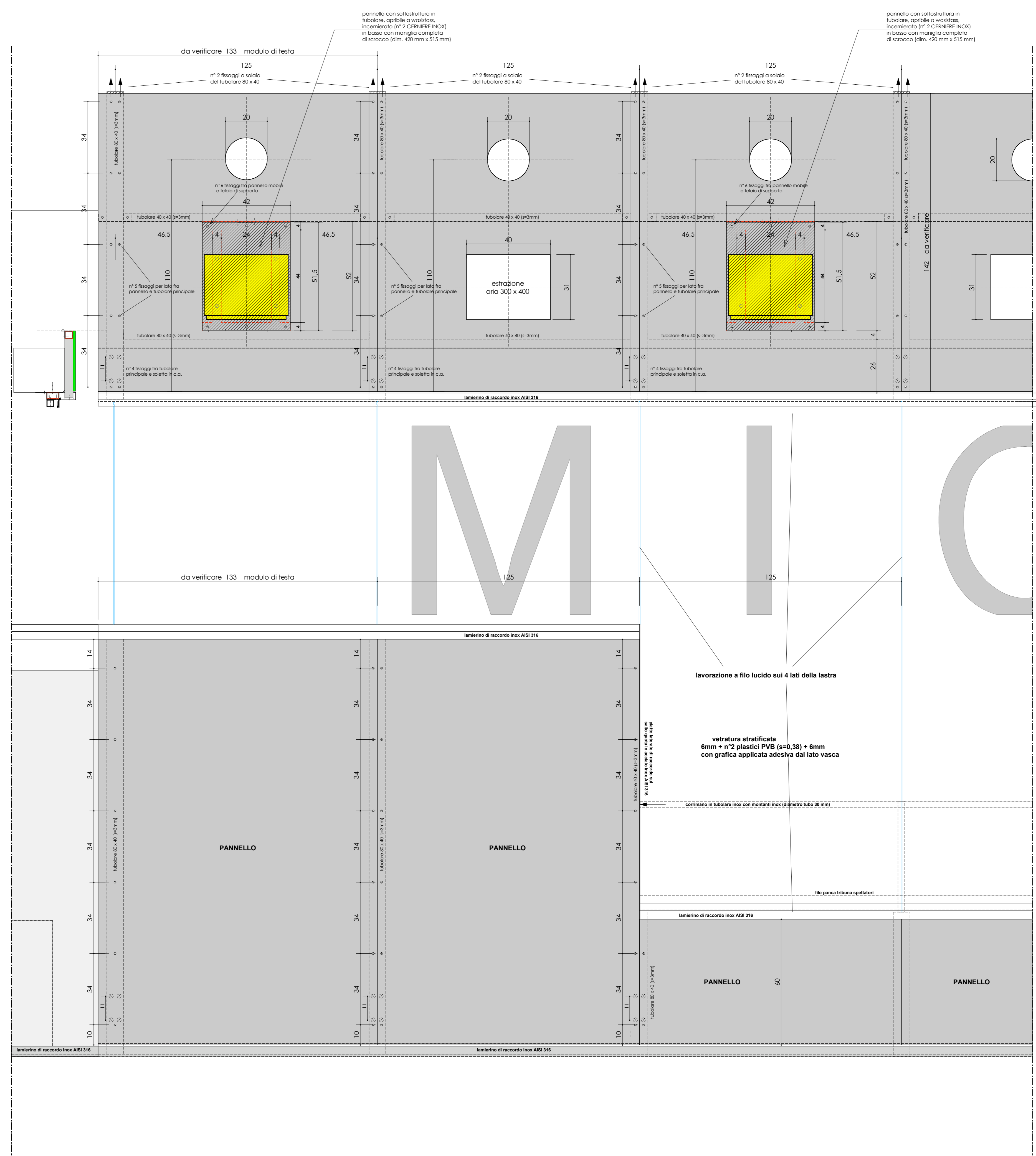
TRIBUNA SPETTATORI PISCINA - PROSPETTO FRONTALE (particolare) - scala 1/10
