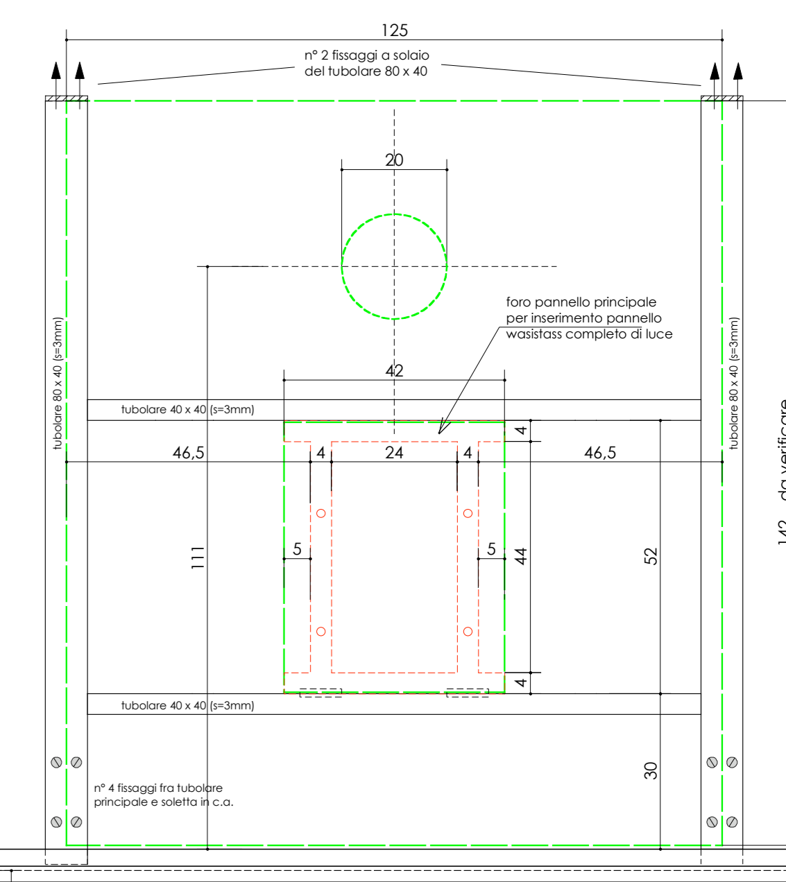
particolare della struttura in ferro zincato di supporto ai pannelli in laminato stratificato
