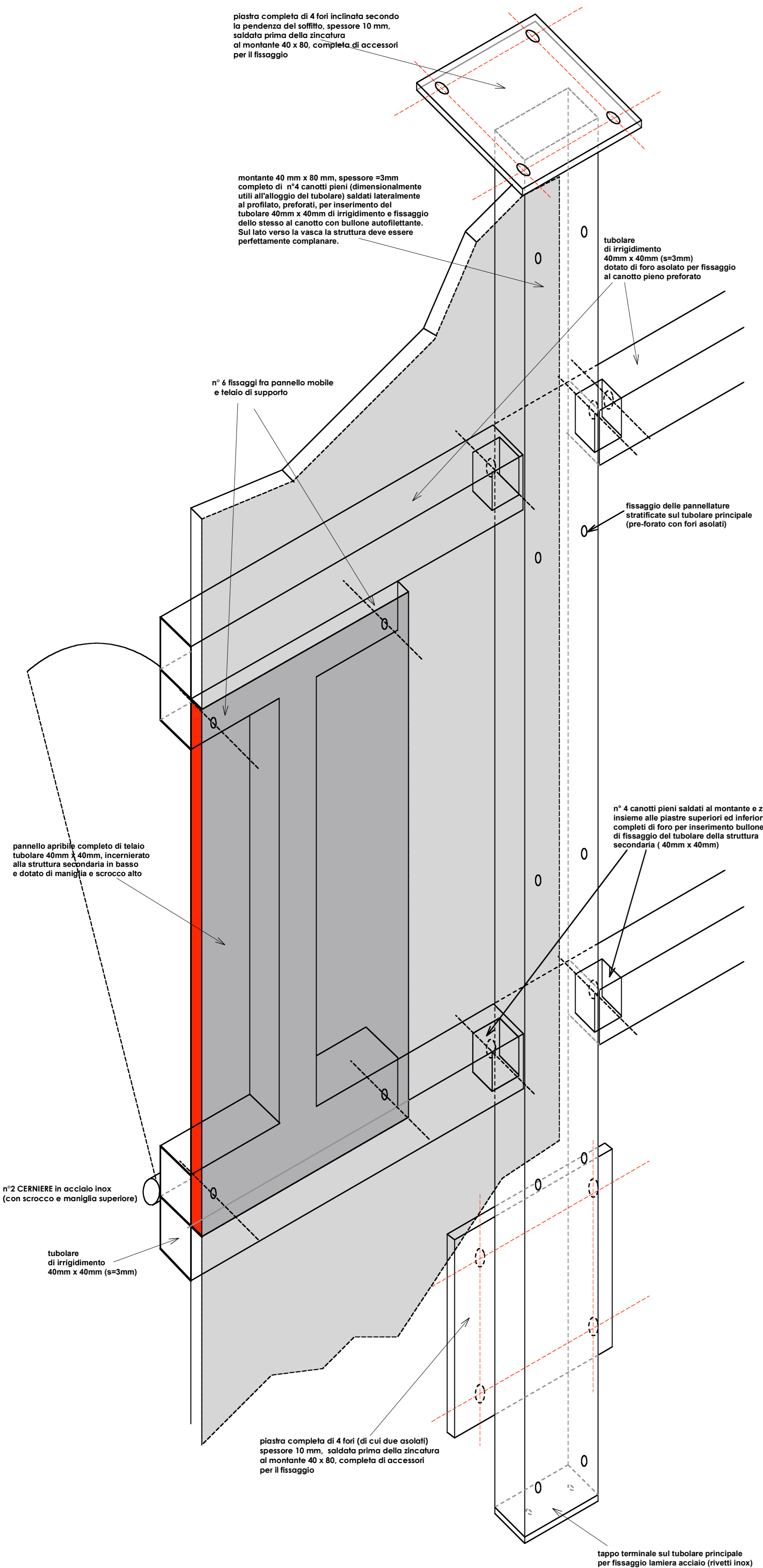
TRIBUNA SPETTATORI PISCINA - STRUTTURA PANNELLATURA (particolare) - scala 1/10
