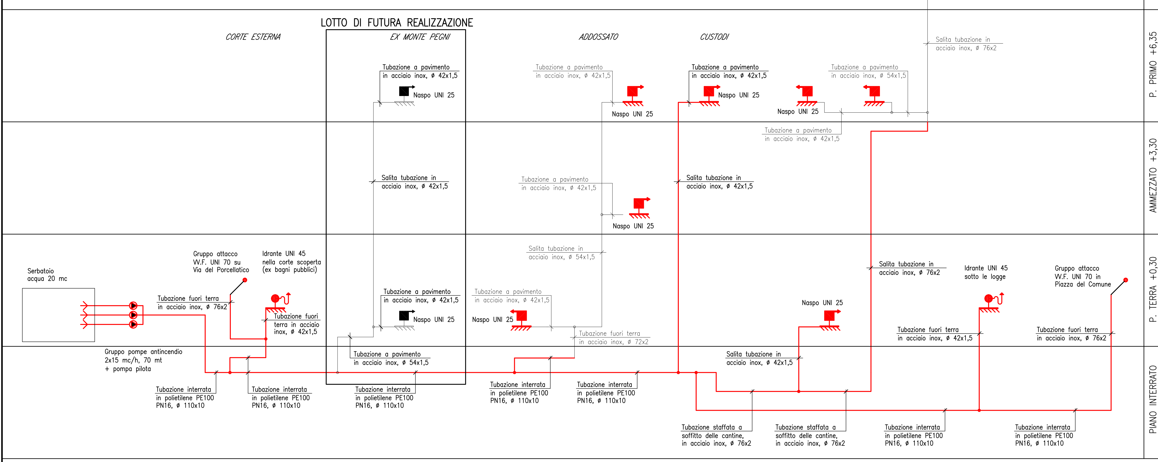
SCHEMA IDRAULICO RETE ANTINCENDIO
