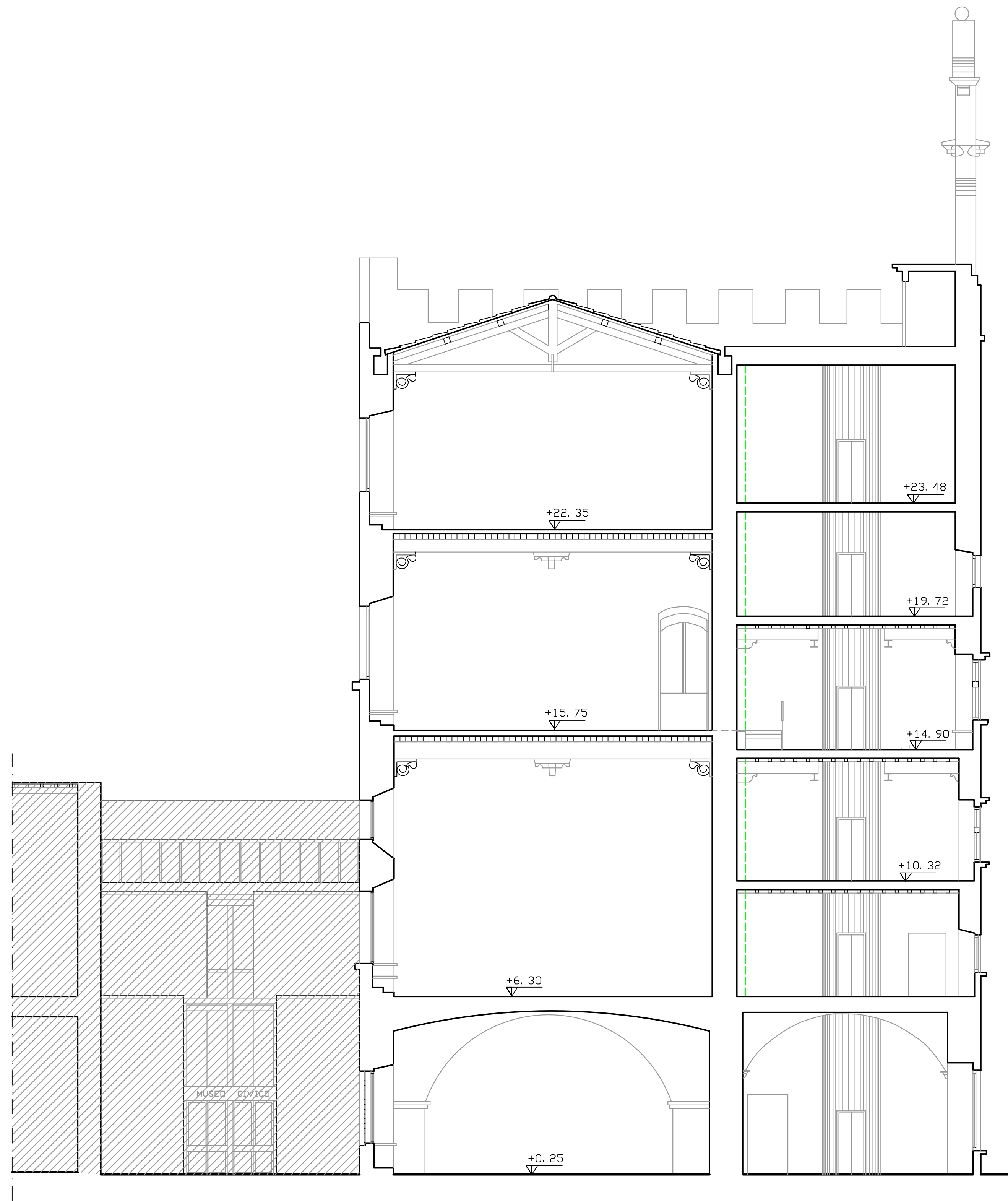
SEZIONE A-A
