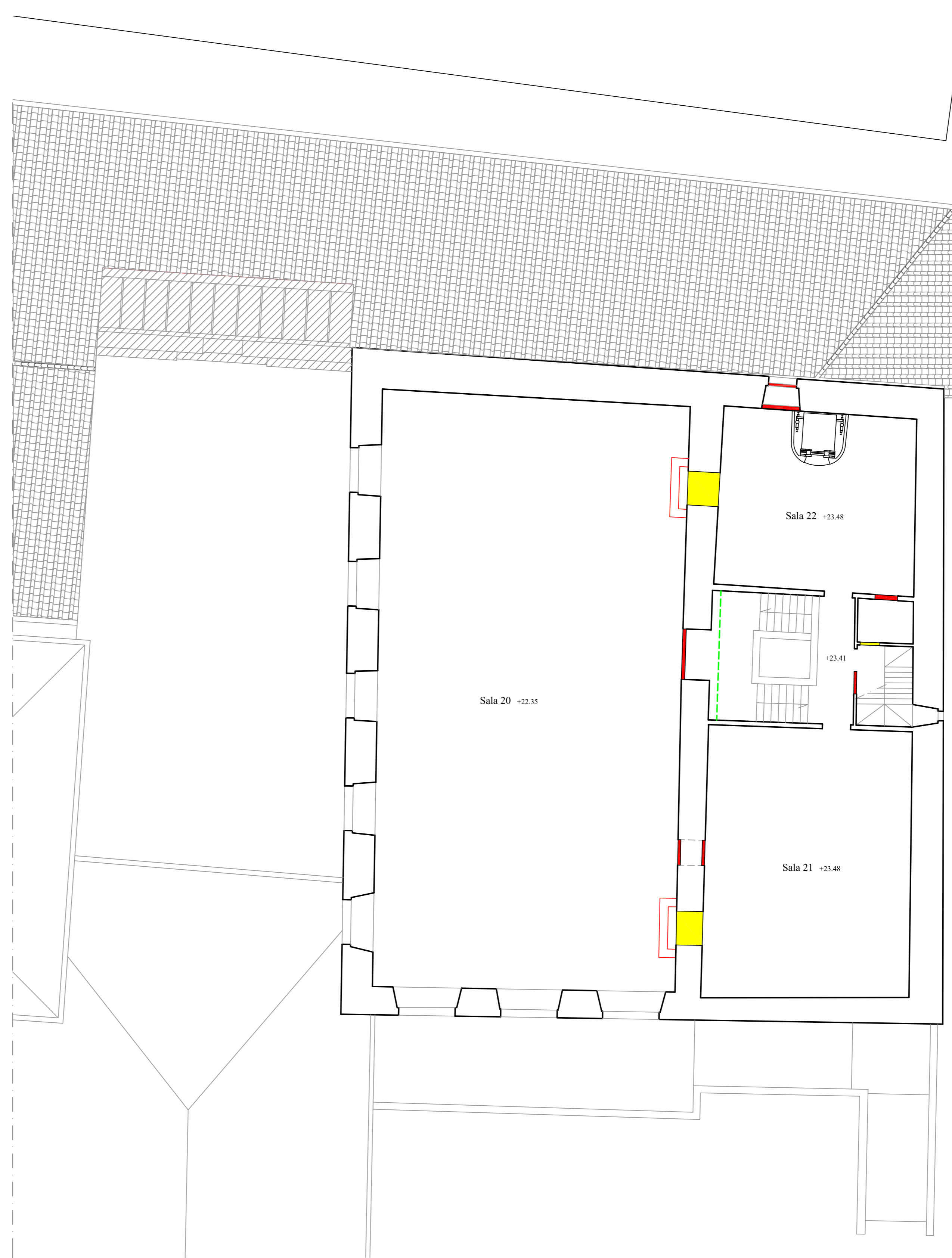
PIANTA A QUOTA +22,35/+23,48
