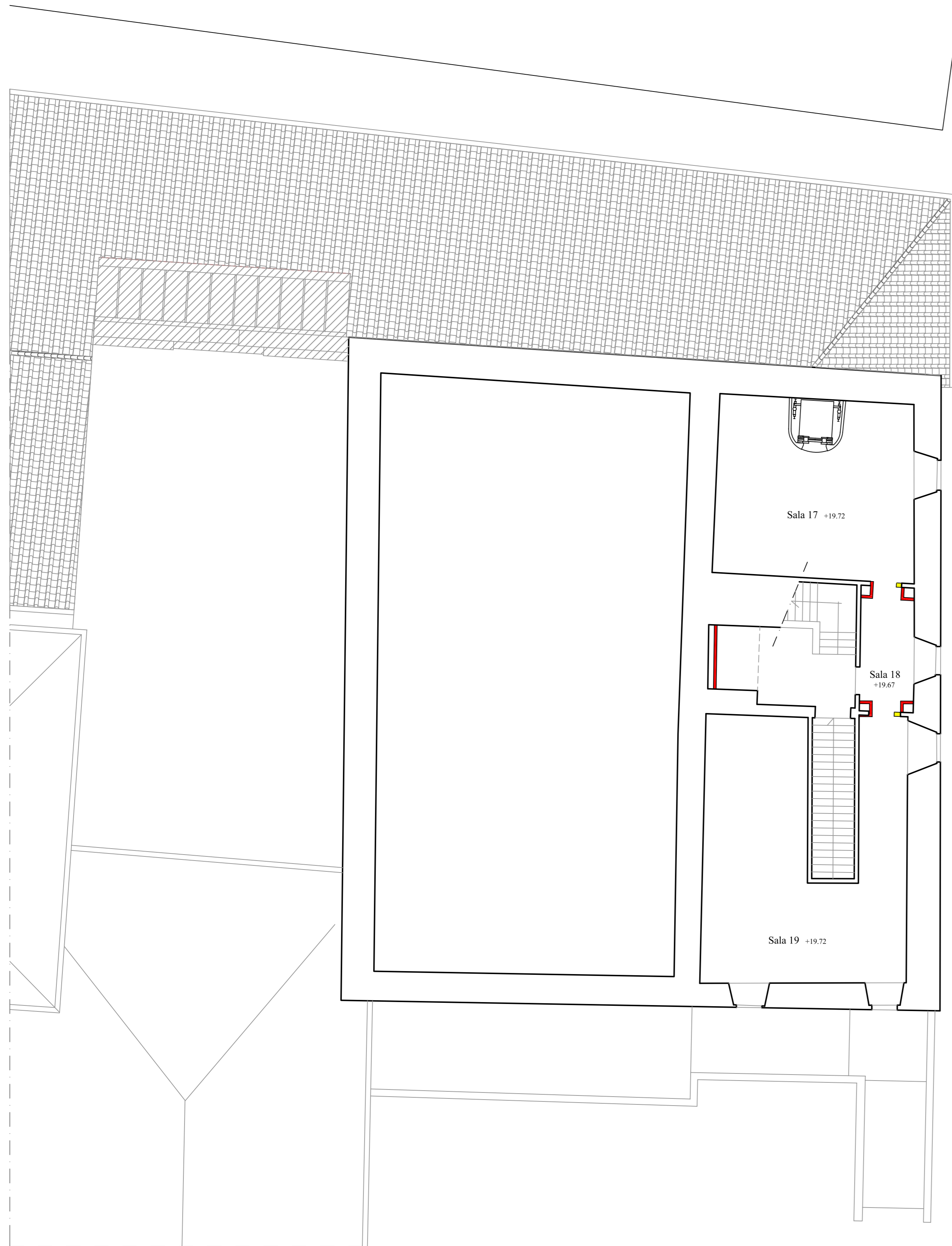
PIANTA A QUOTA +19,72
