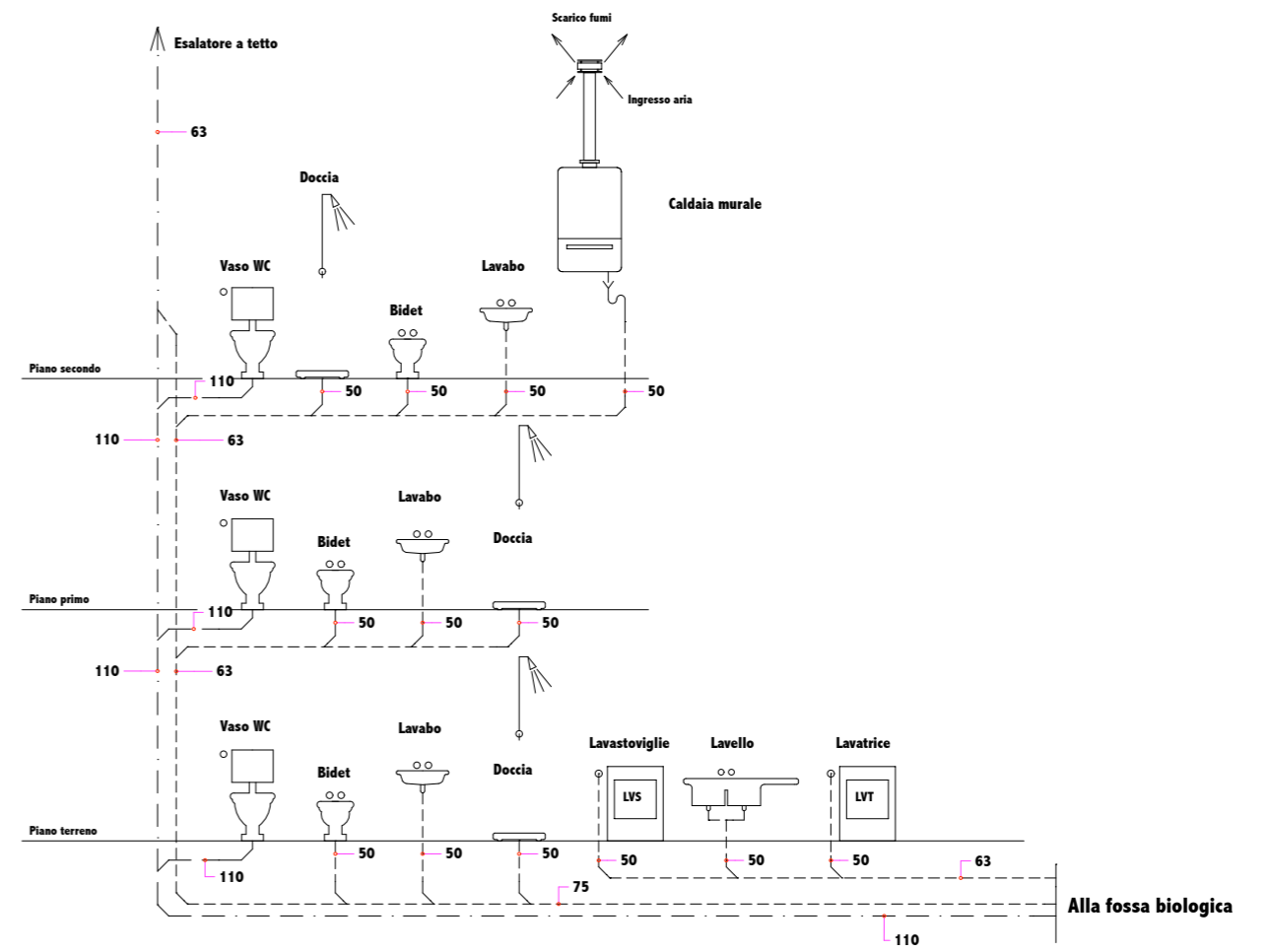
Schema idraulico dei collegamenti
